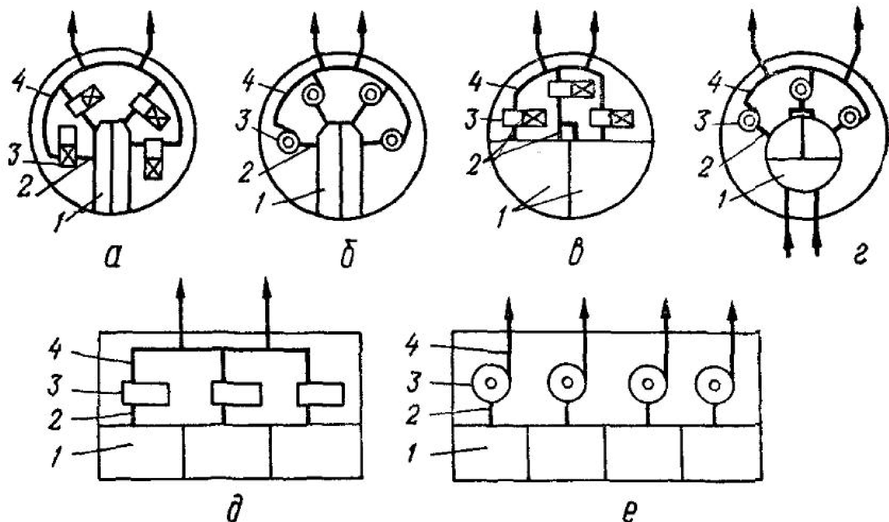
Рис. 43. Схемы размещения оборудования в совмещенных насосных станциях I подъема:
