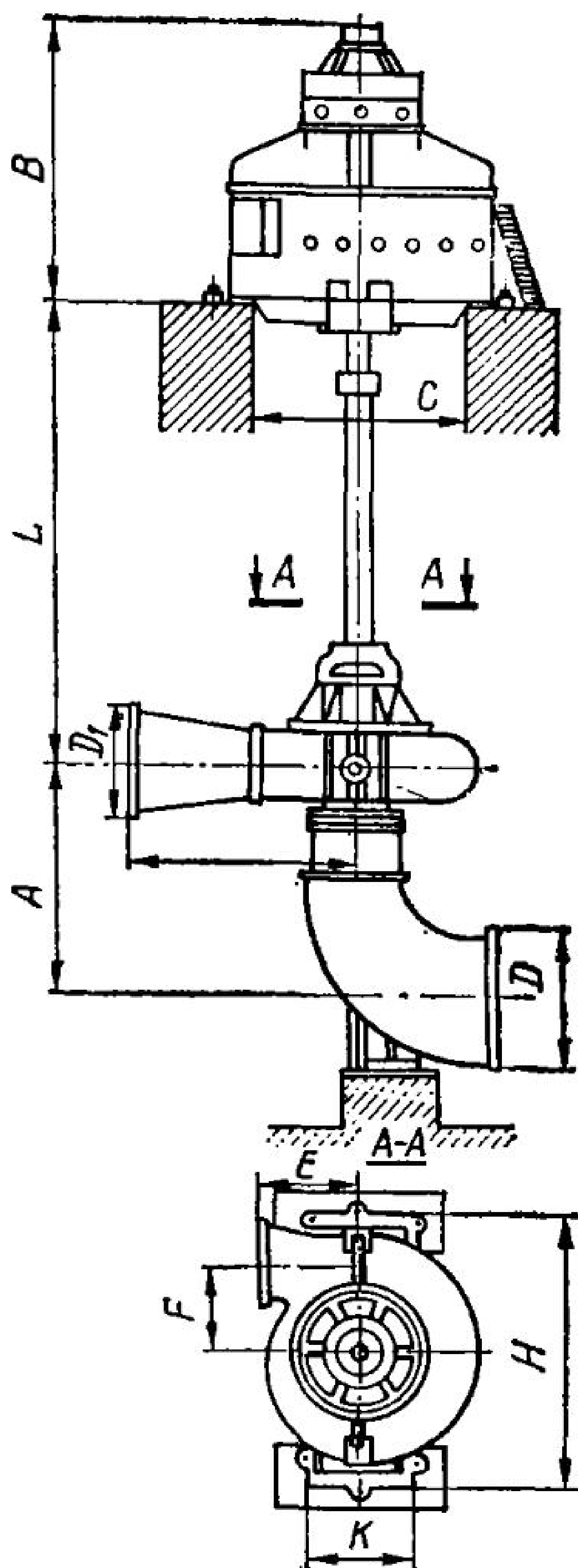
Рис. 6. Габаритные размеры вертикальных насосов типа В (СДВ) с электродвигателями
