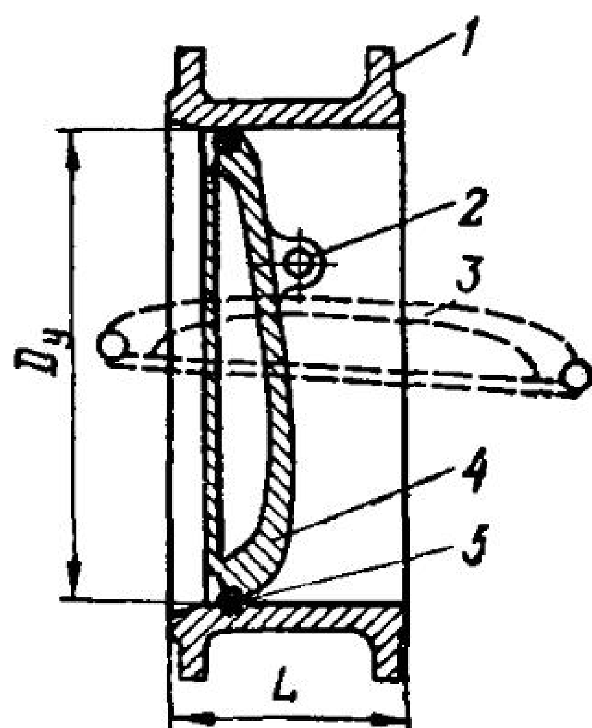
Рис. 20. Клапан обратный поворотный безударный:
