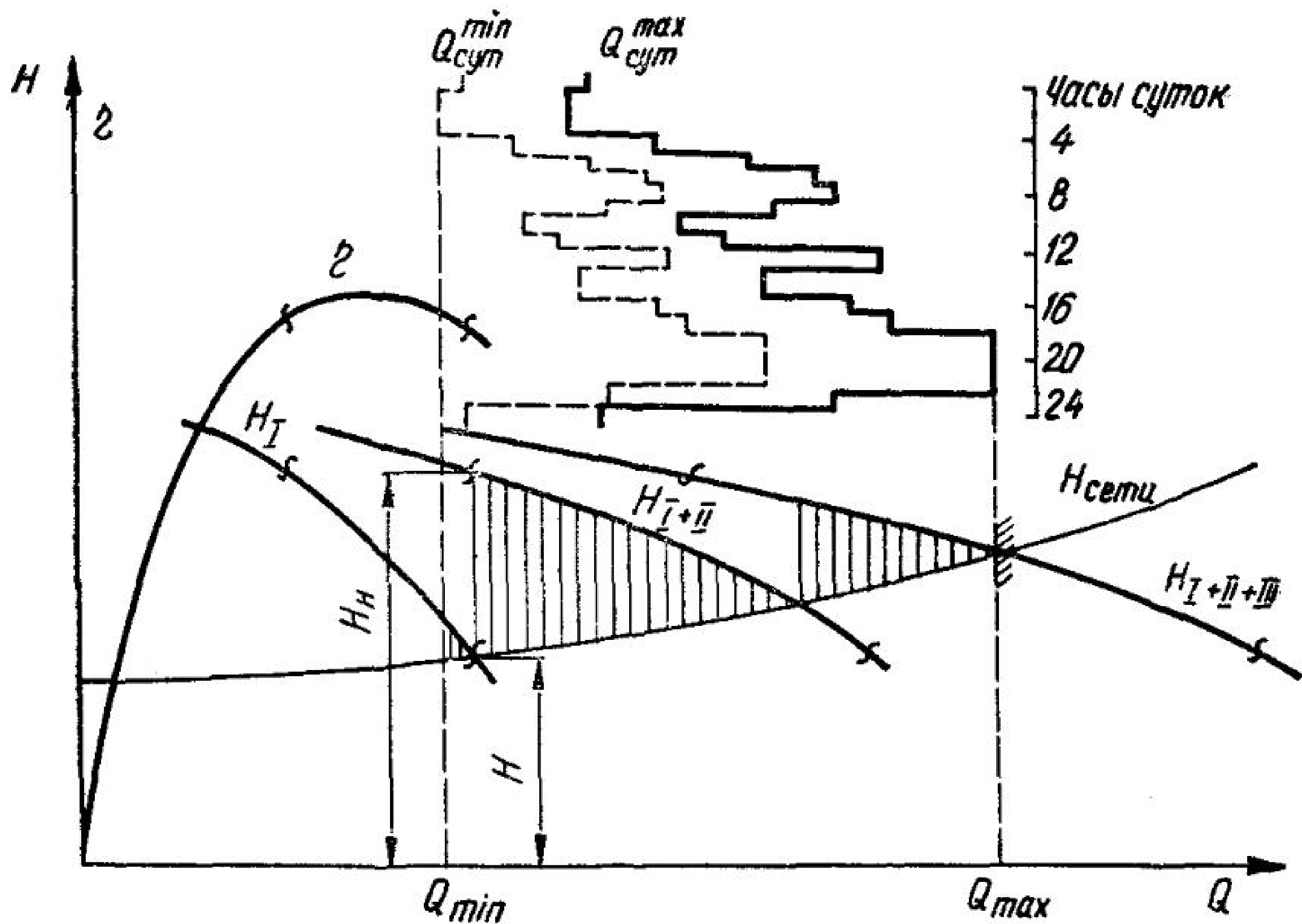
Рис. 50. График работы насосов II подъема в безбашенной системе водопровода
