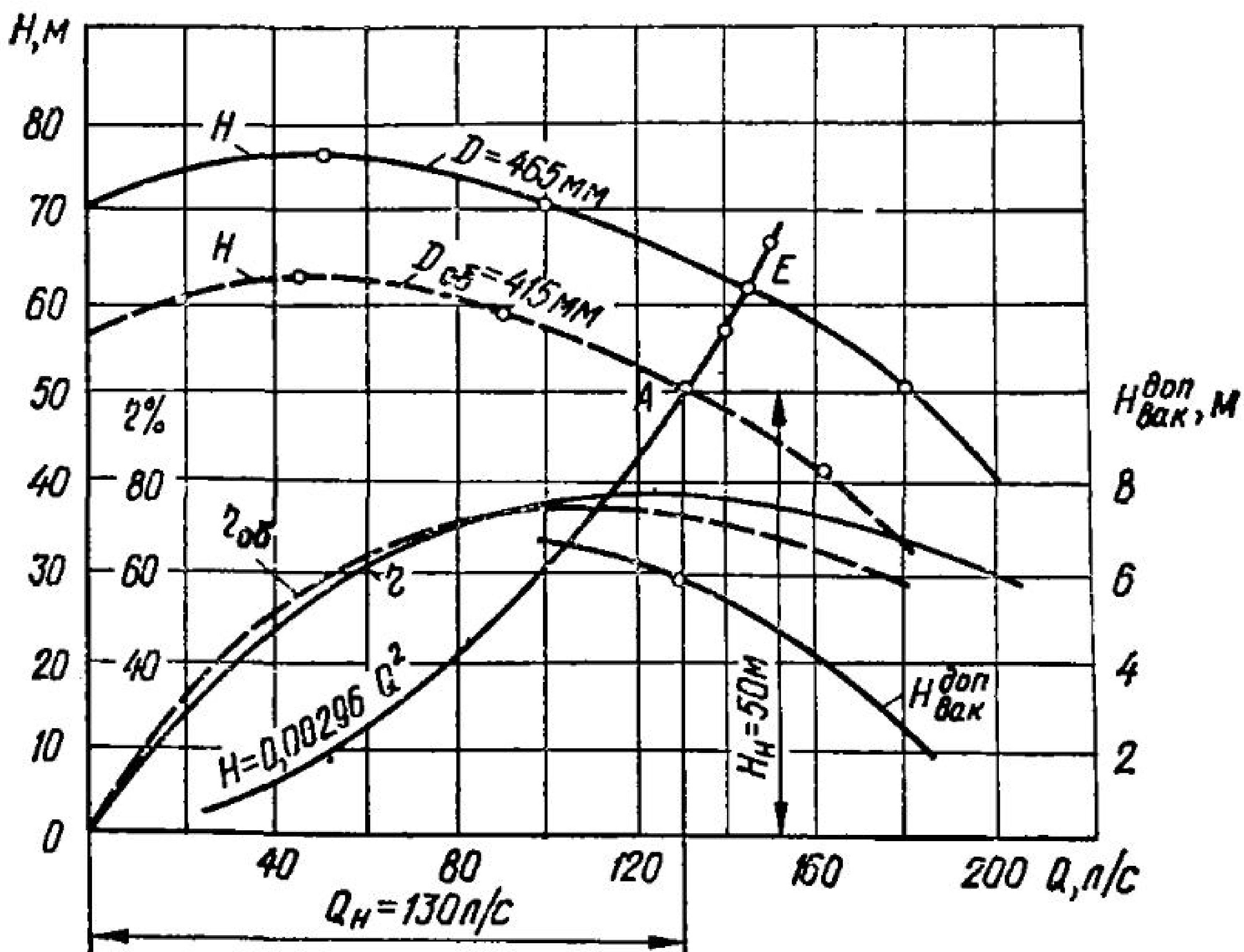
Рис. 10. Построение характеристик насоса с обточенным рабочим колесом
