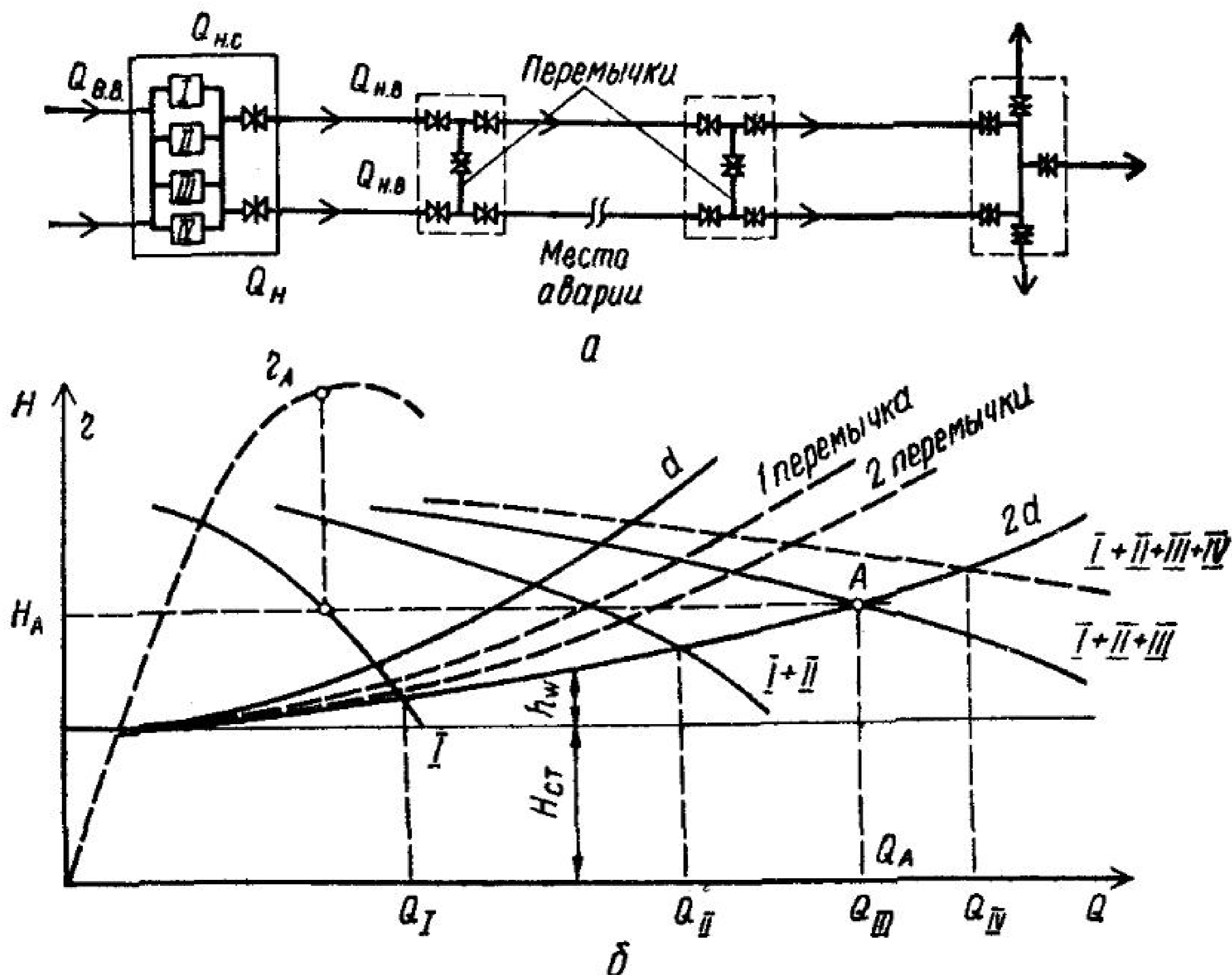
Рис. 24. Параллельная работа 4-х насосов на два водовода с перемычками:
