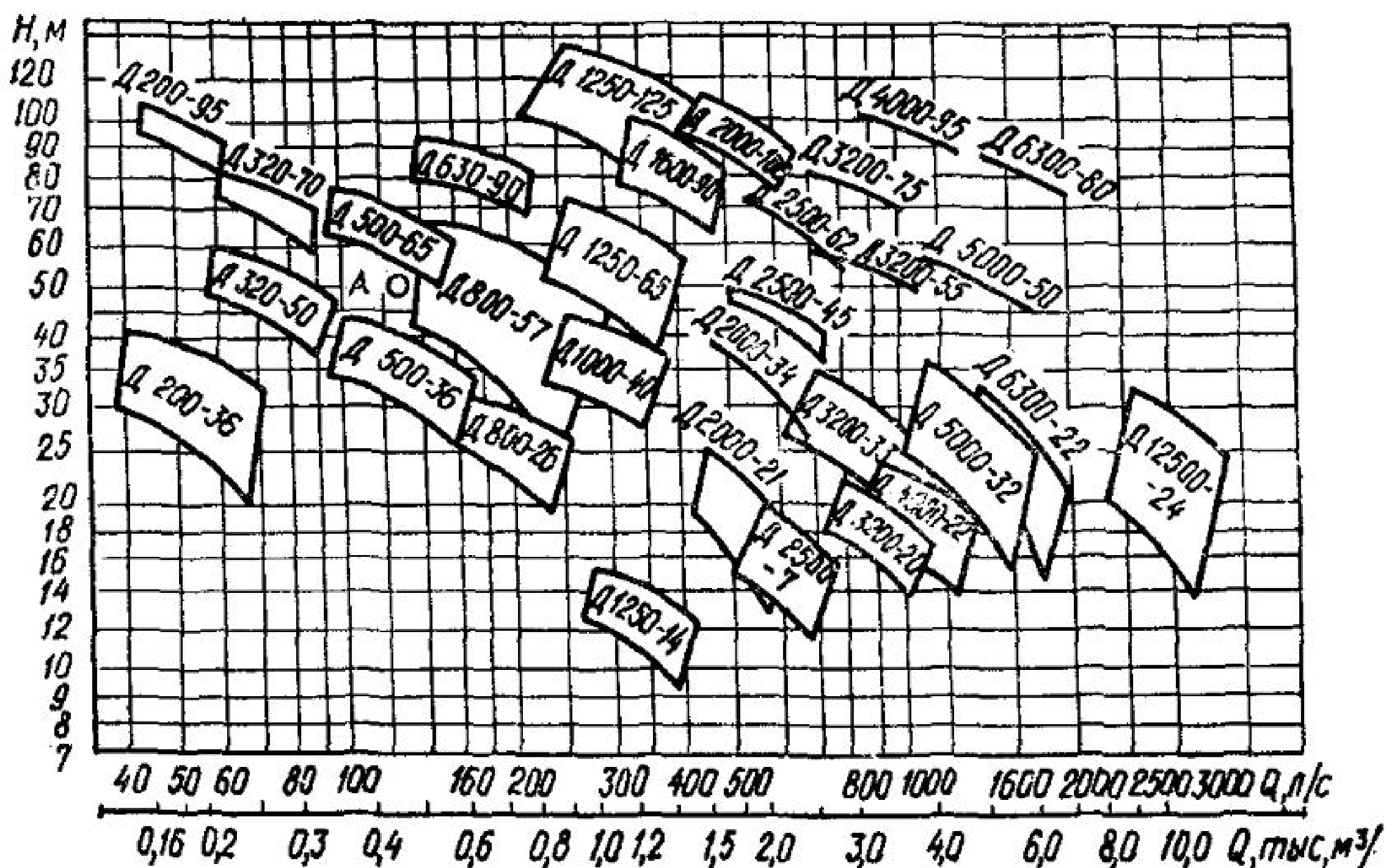
Рис. 5. Сводный график полей насосов типа Д
