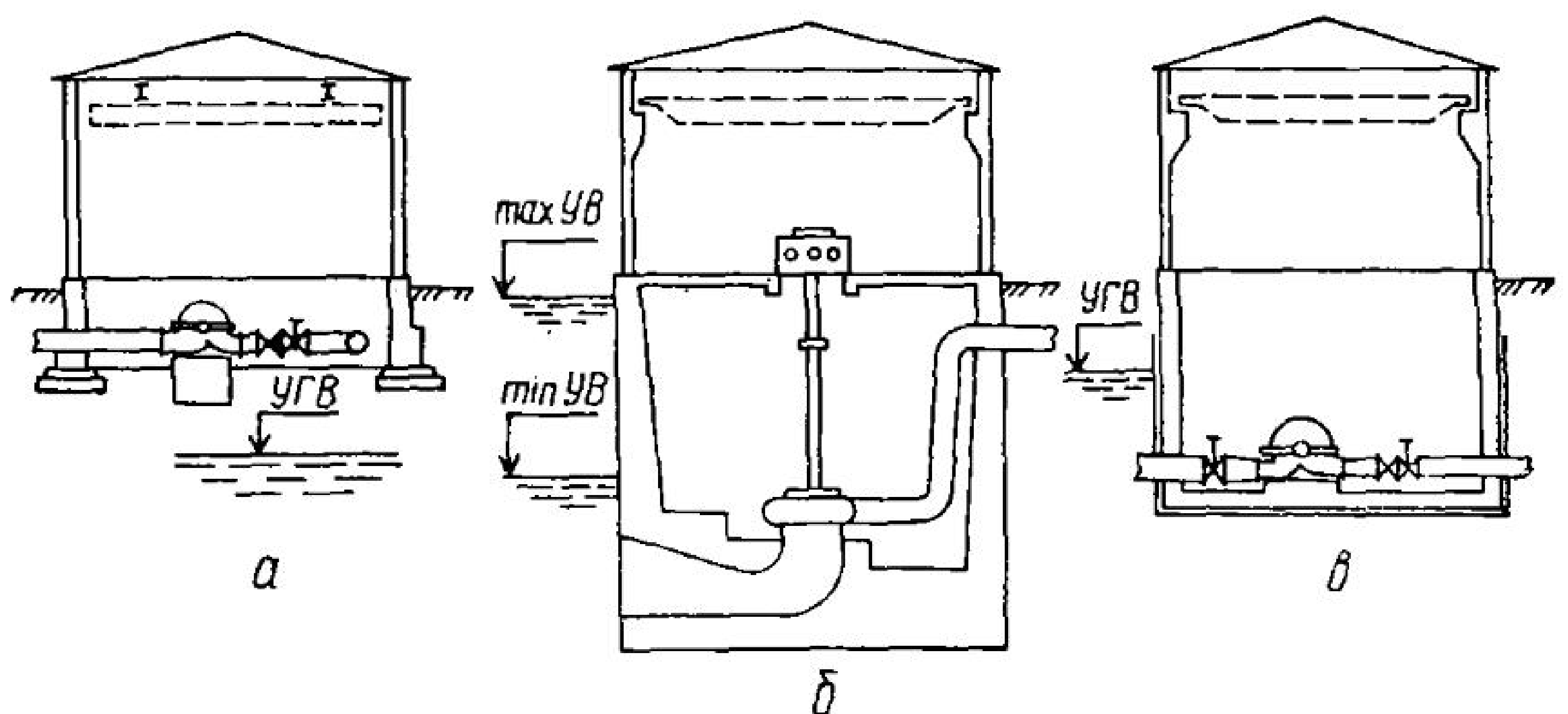
Рис. 33. Типы конструкций подземной части насосных станций: а — с отдельными фундаментами под оборудование и строительные конструкции; б — блочная; в — камерная
