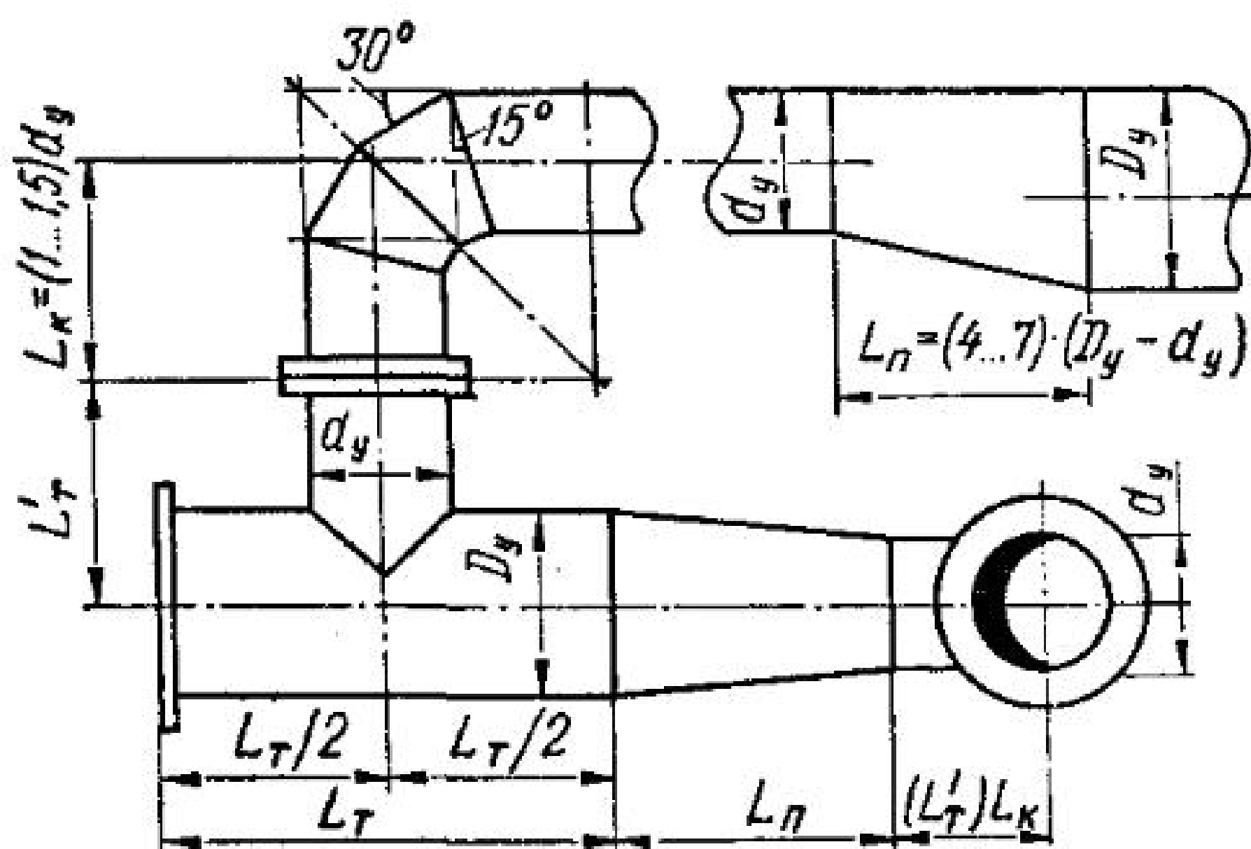
Рис. 15. Сварные фасонные части
