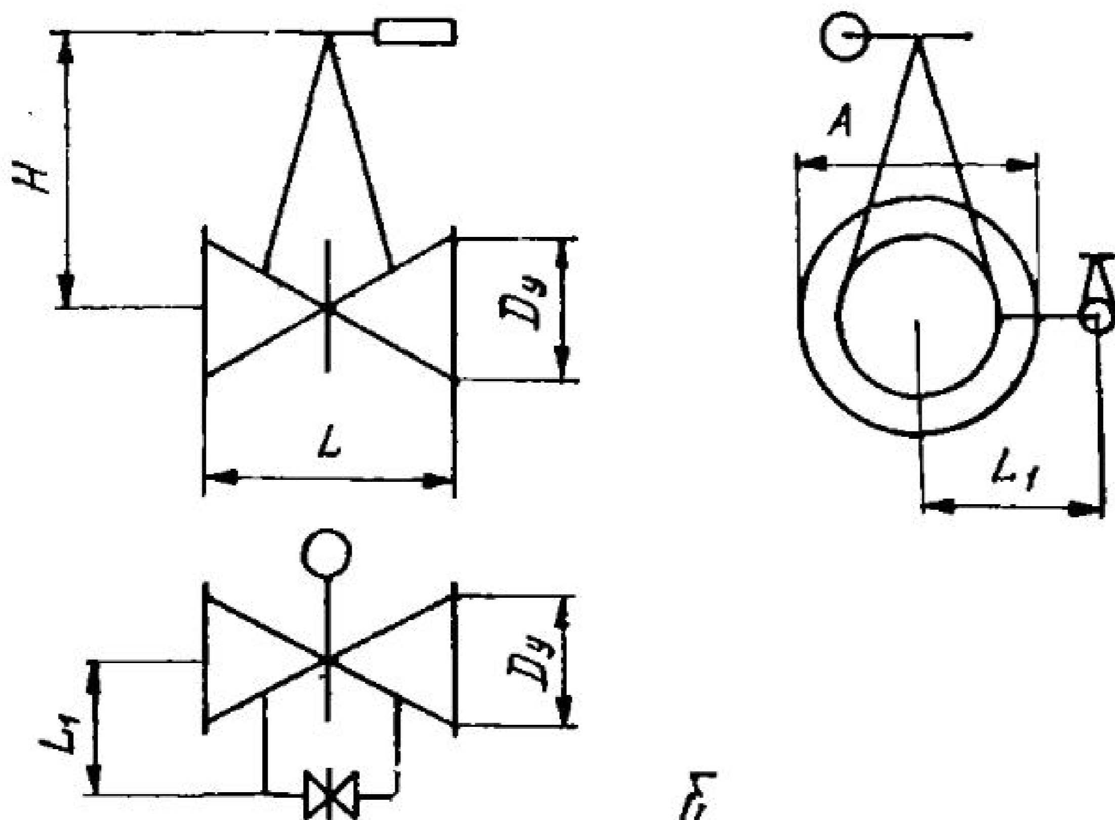
Рис. 18. Задвижка с электроприводом:
