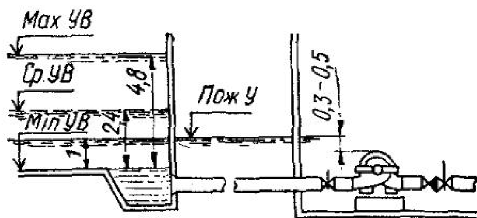
Рис. 55. Схема высотного расположения насосов на станции II подъема
