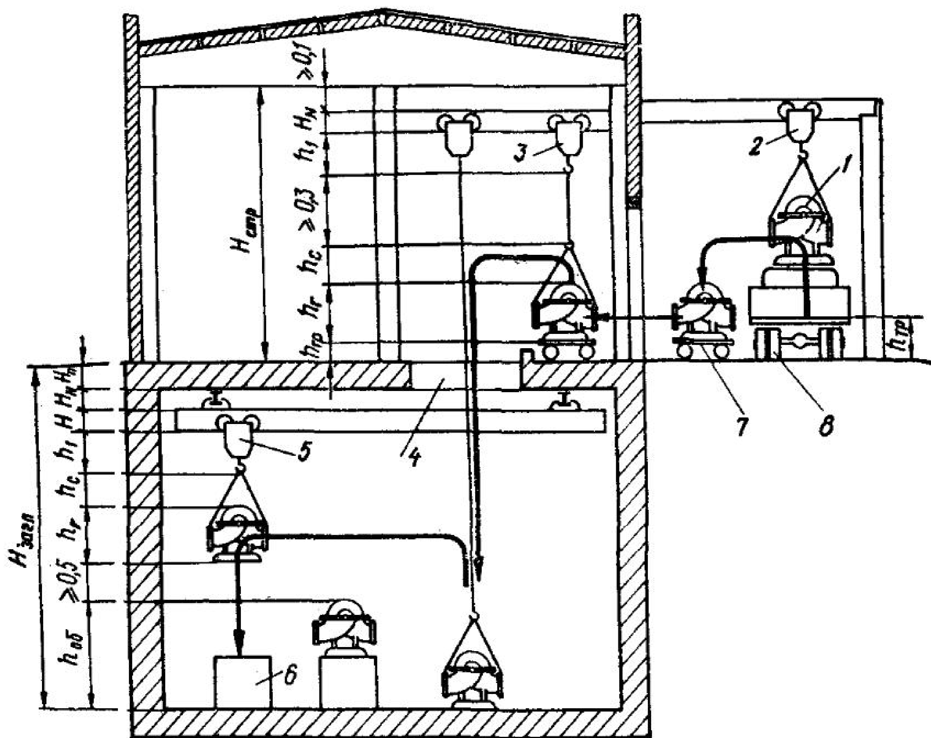
Рис. 19. Схема подъемно-транспортных операций в заглубленных и насосных станциях:
