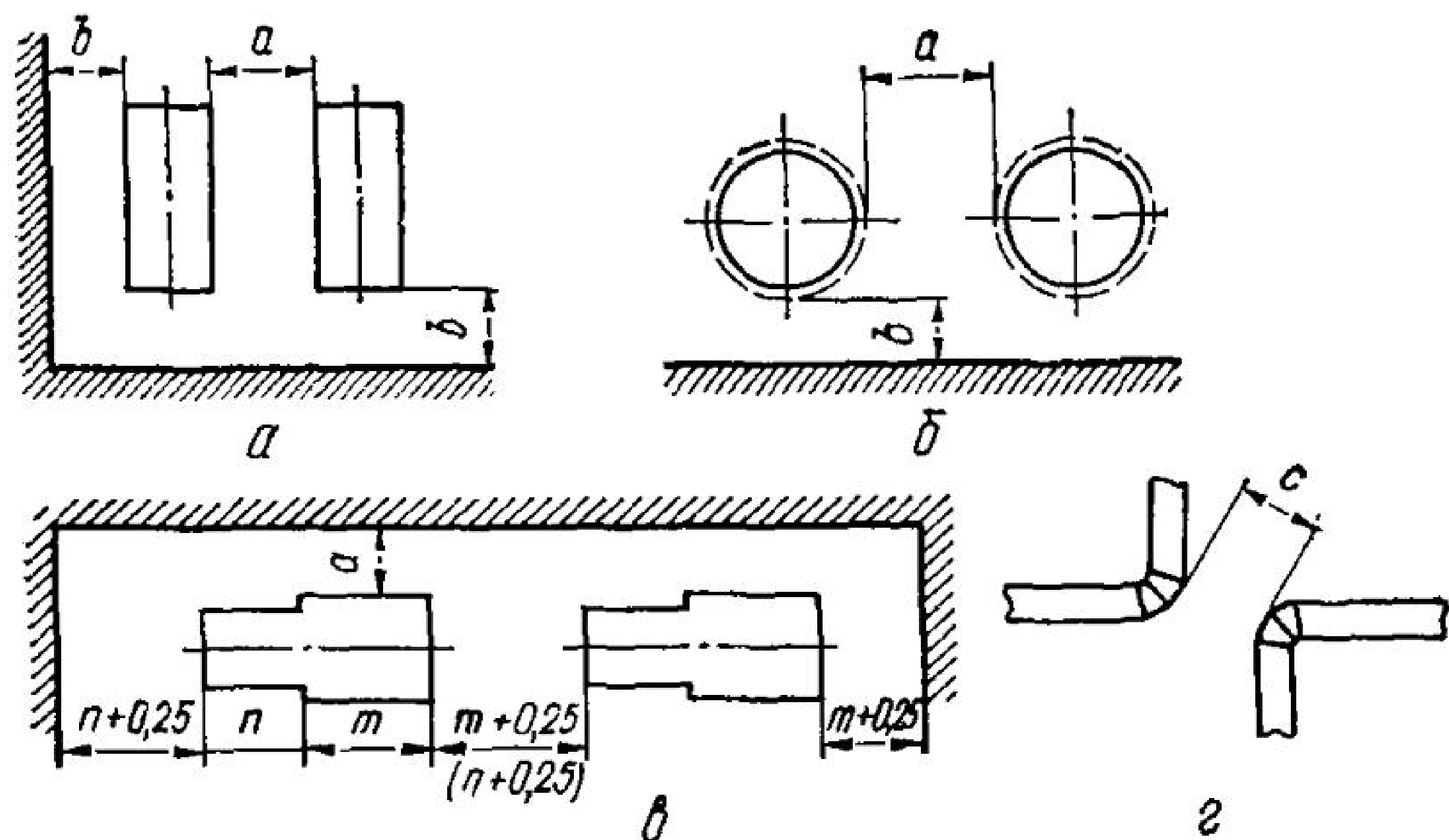
Рис. 13. Схема к определению ширины проходов в машинном зале:
