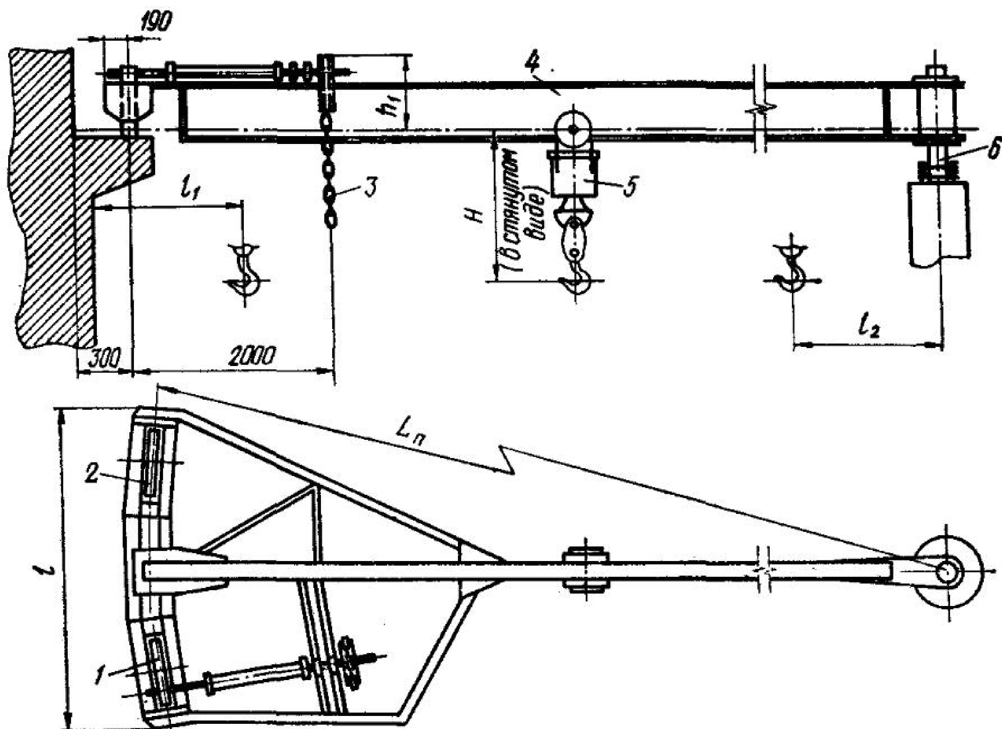
Рис. 32. Кран мостовой радиальный:
