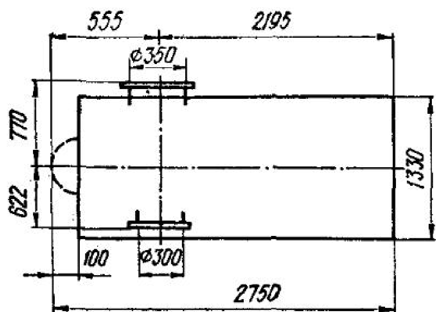
Рис. 45. Монтажное пятно насоса Д1250-65 с электродвигателем
