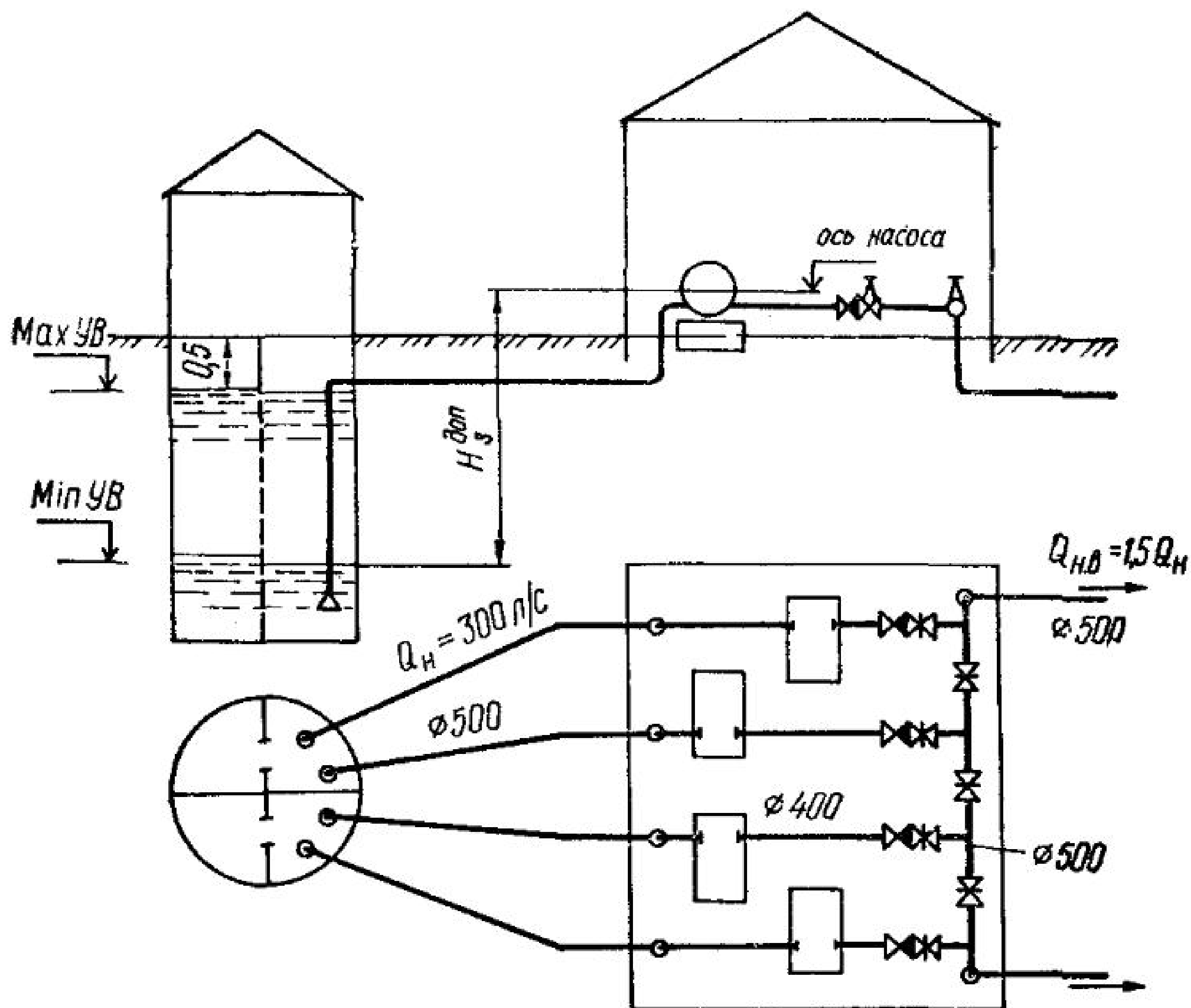
Рис. 44. Схема размещения насосов, трубопроводов и арматуры в насосной станции I подъема
