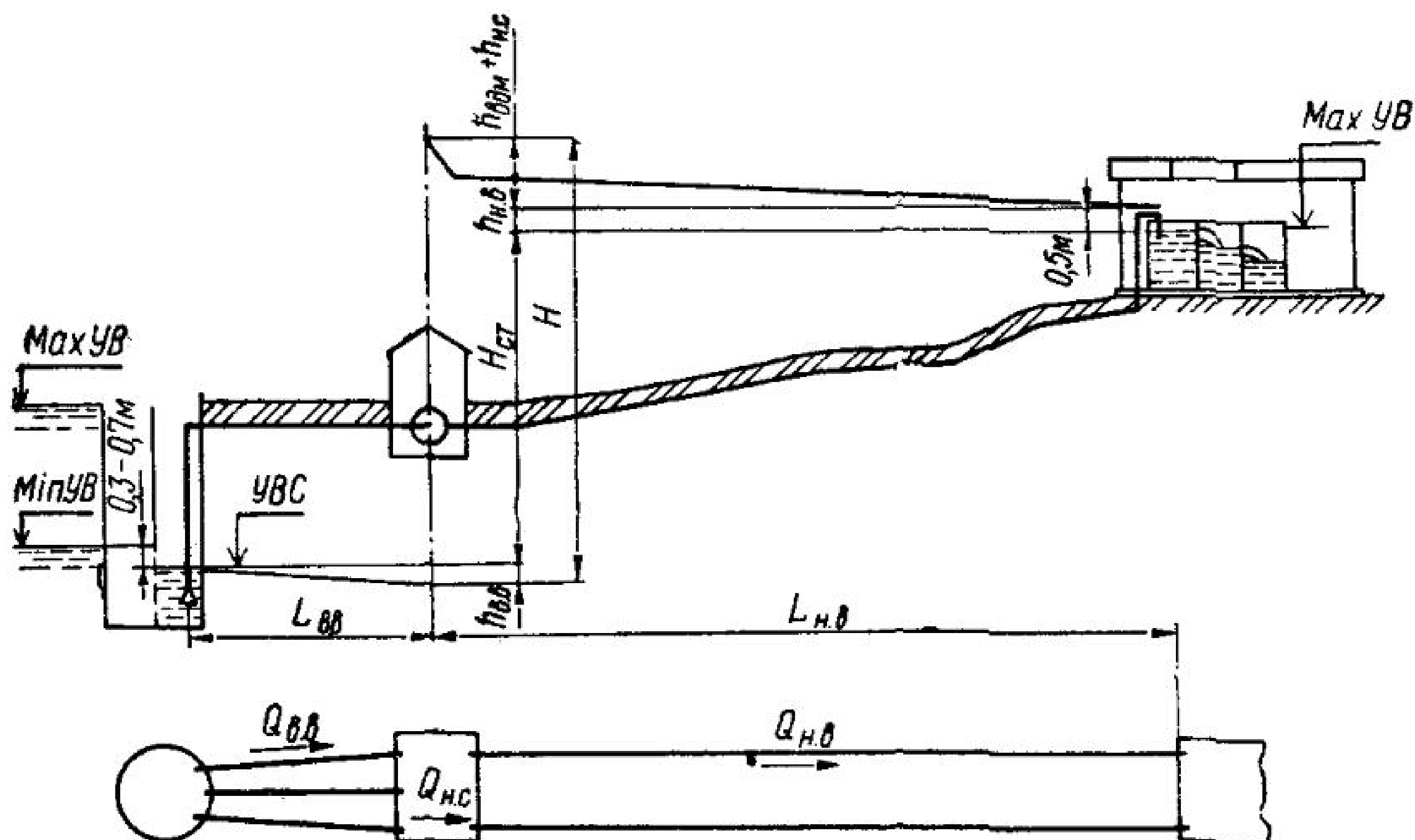
Рис. 40. К определению расчетного напора насосов I подъема: УВС — уровень воды в водоприемно-сеточном колодце
