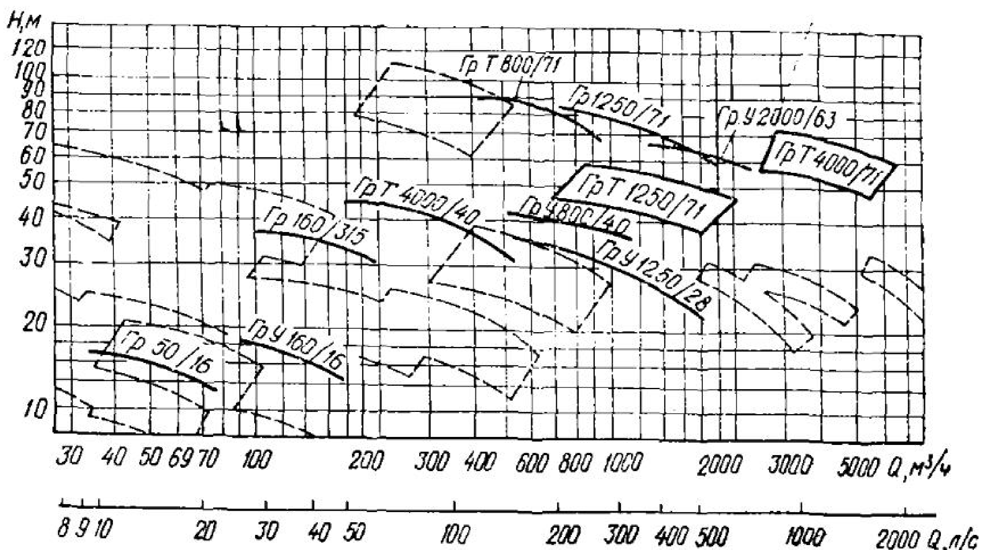
Рис. 9. Сводный график полей насосов типа Гр
