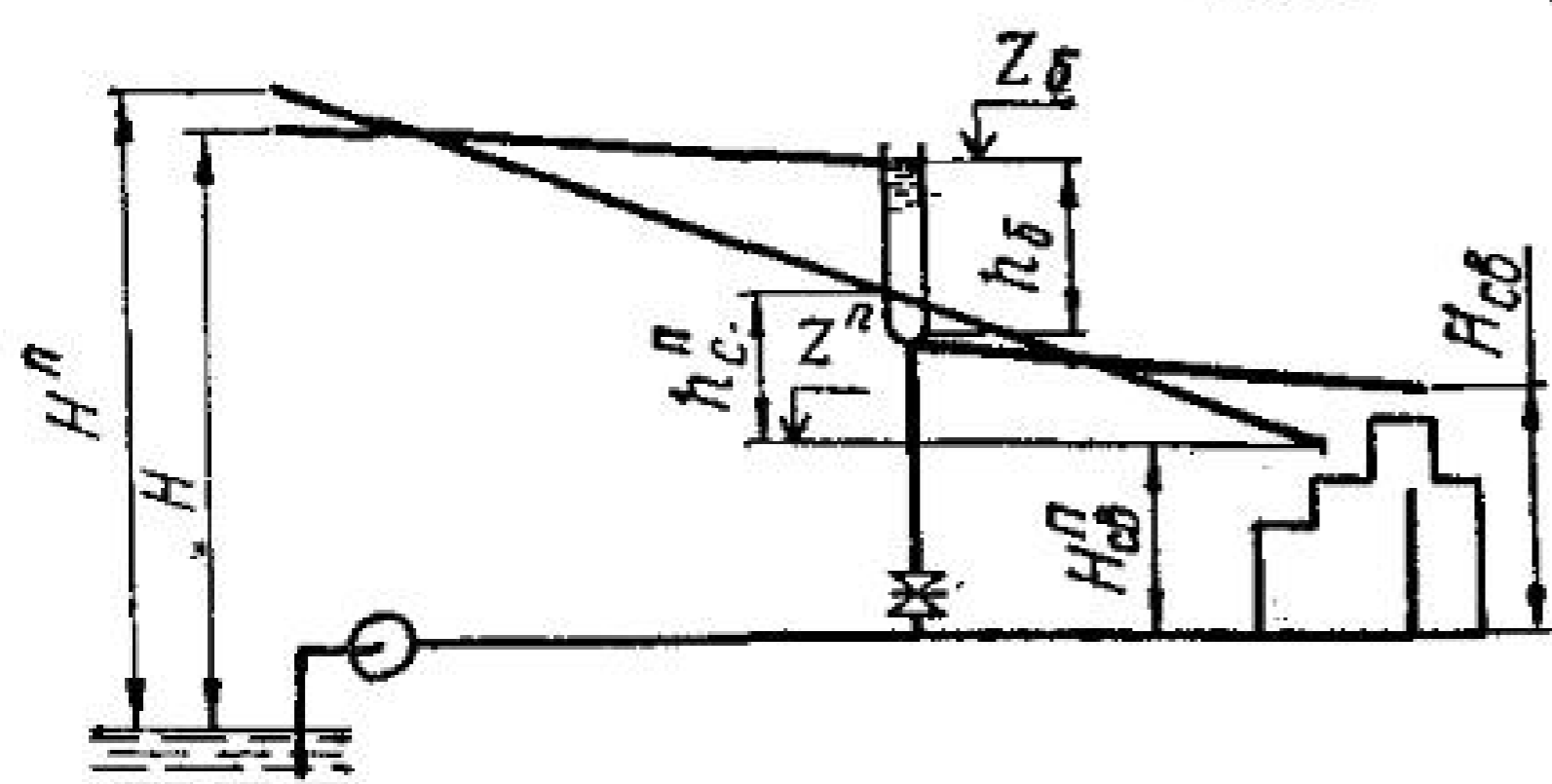
Рис. 53. Схема отключения водонапорной башни при пожаре
