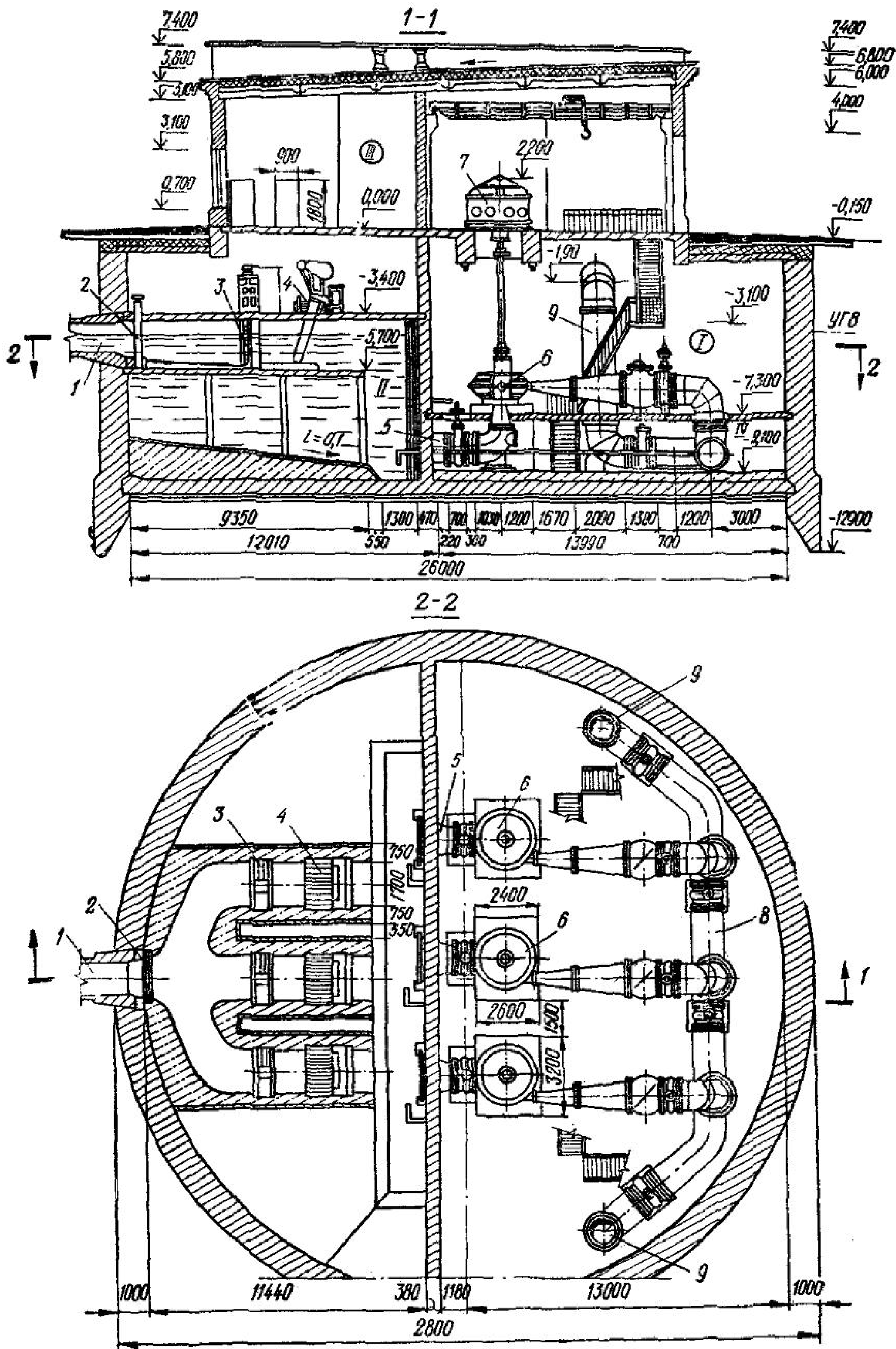
Рис. 61. Насосная станция водоотведения с вертикальными насосами и механизированными решетками:
