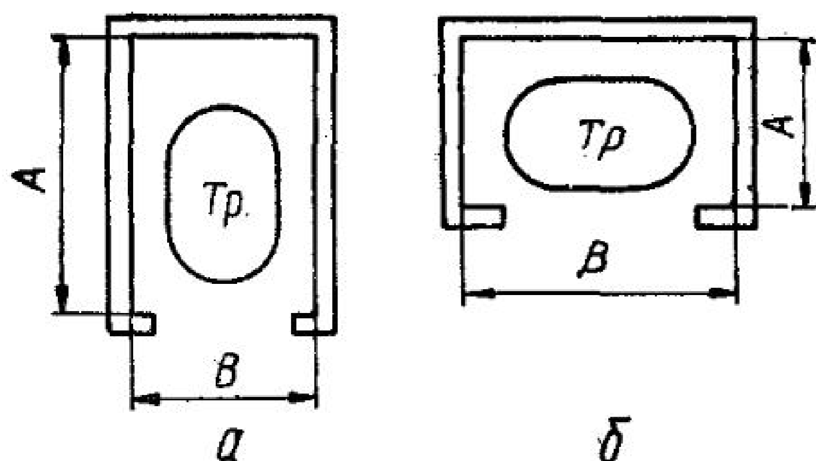
Рис. 37. Габариты трансформаторных камер:
