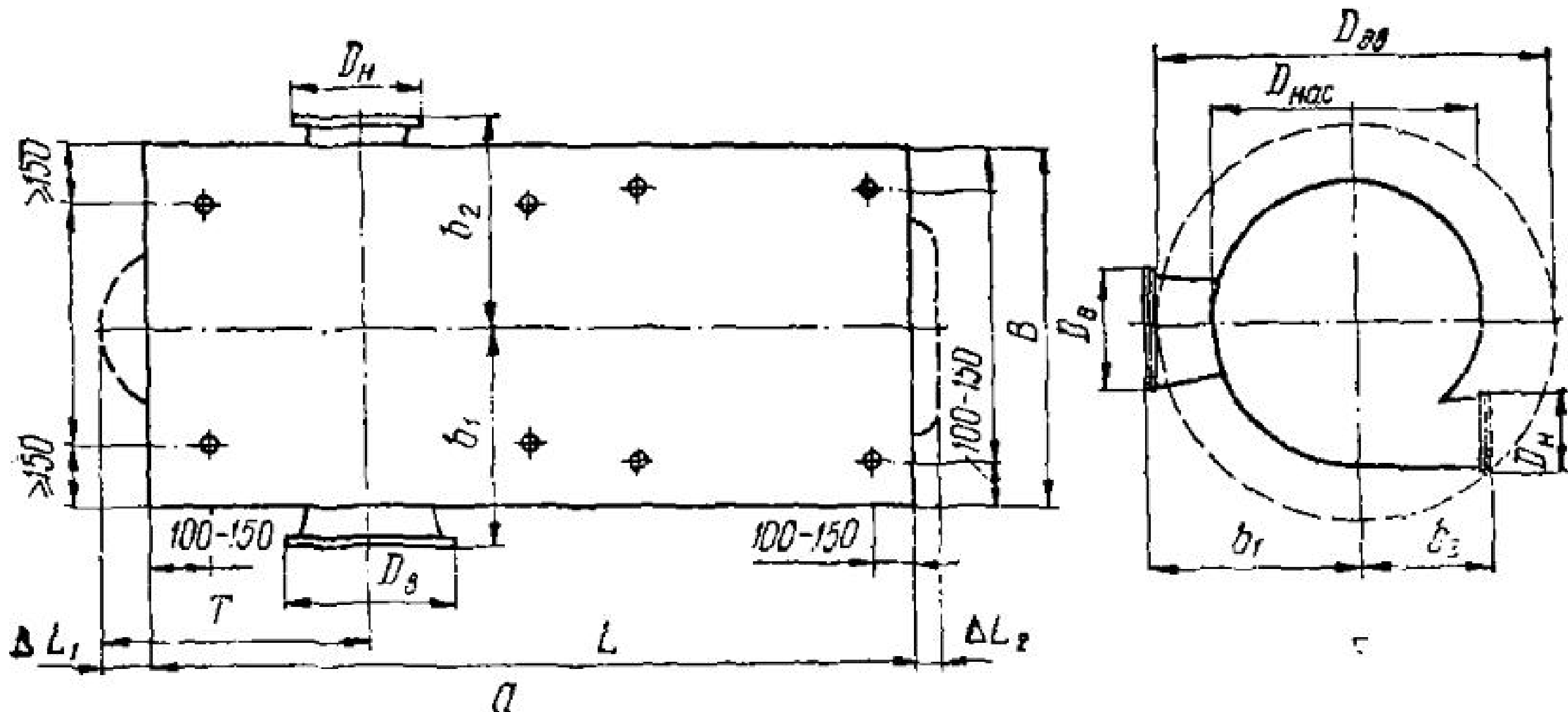
Рис. 11. Монтажные пятна насосов: а — горизонтального; б — вертикального
