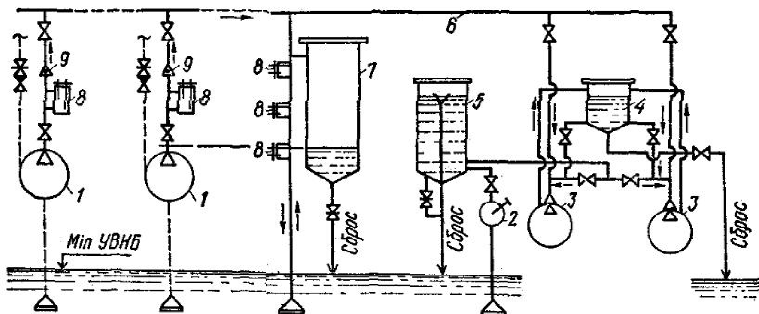
Рис. 27. Схема заливки основных насосов при помощи вакуум-котла:
