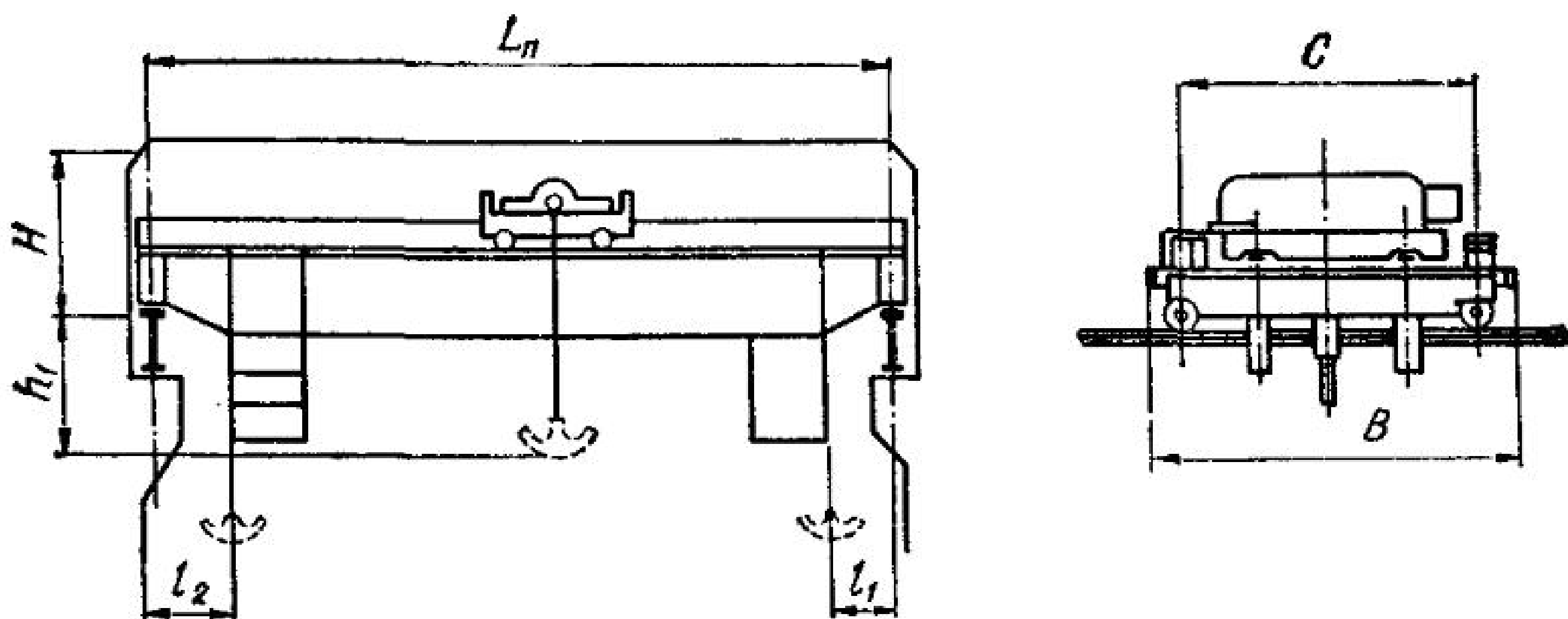
Рис. 31. Кран мостовой электрический грузоподъемностью 5—30 т
