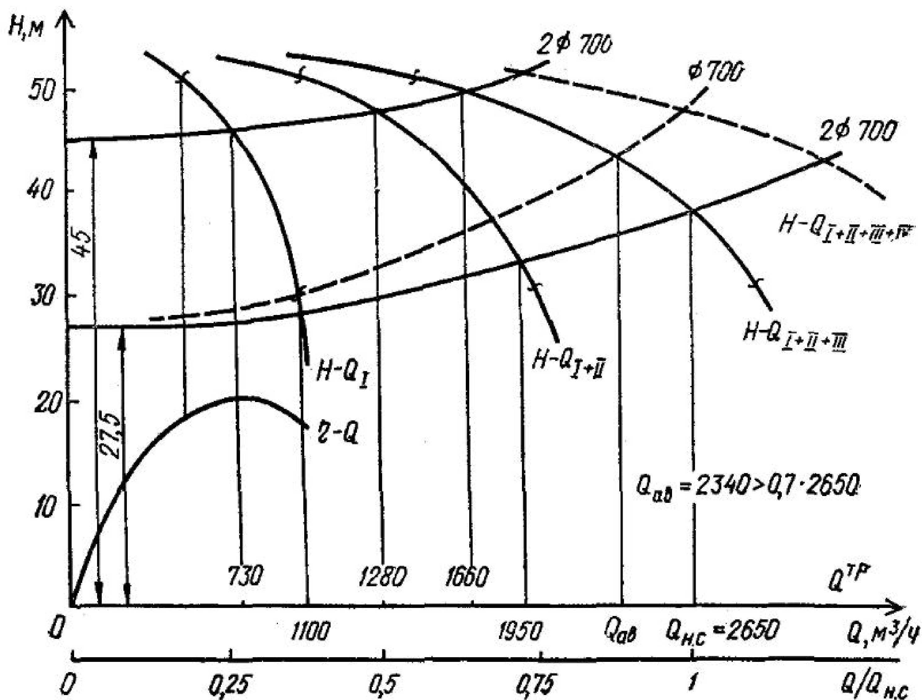
Рис. 52. График работы насосов II подъема в системе с контр-резервуаром
