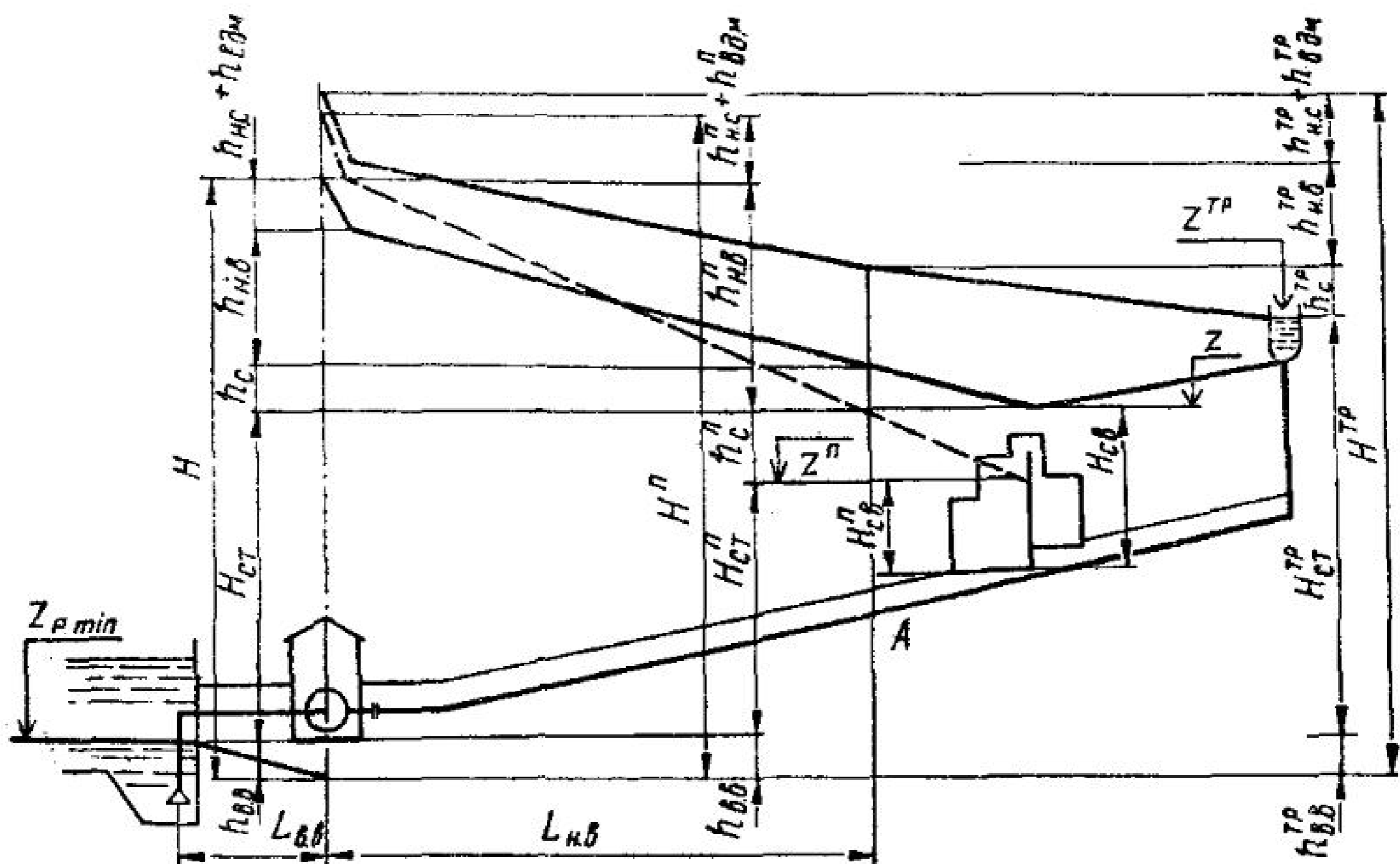
Рис. 51. Схема к определению напора насосов II подъема в системе с контррезервуаром
