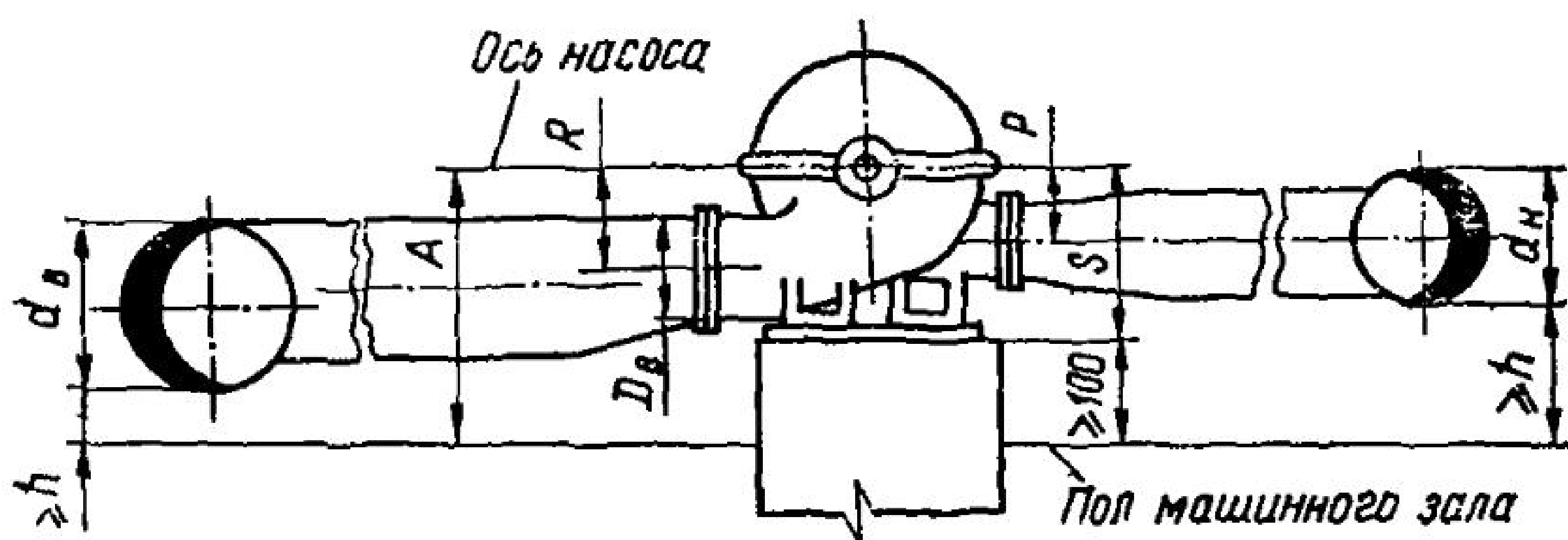
Рис. 12. Схема к определению возвышения фундамента насоса над полом
