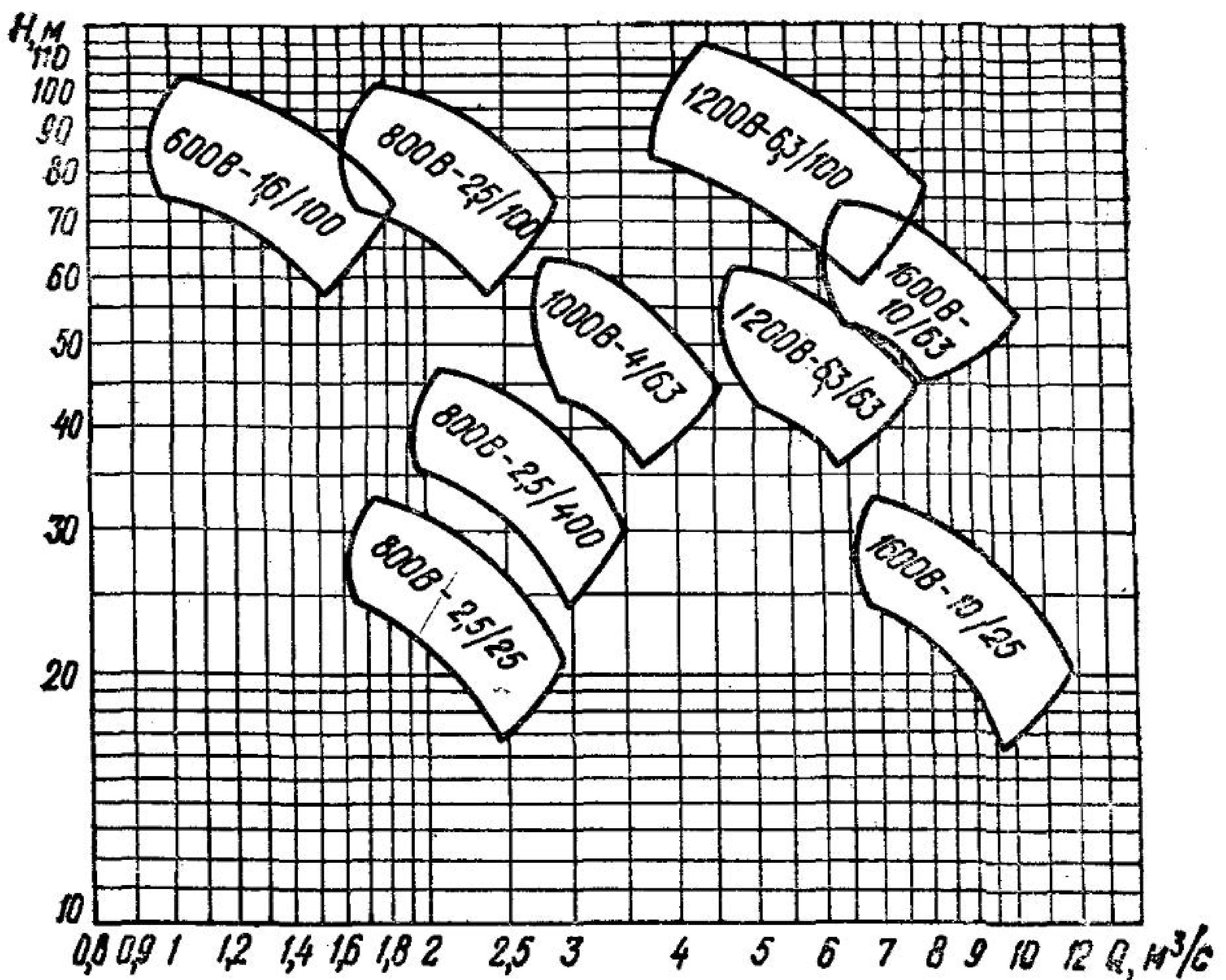
Рис. 7. Сводный график полей насосов типа В
