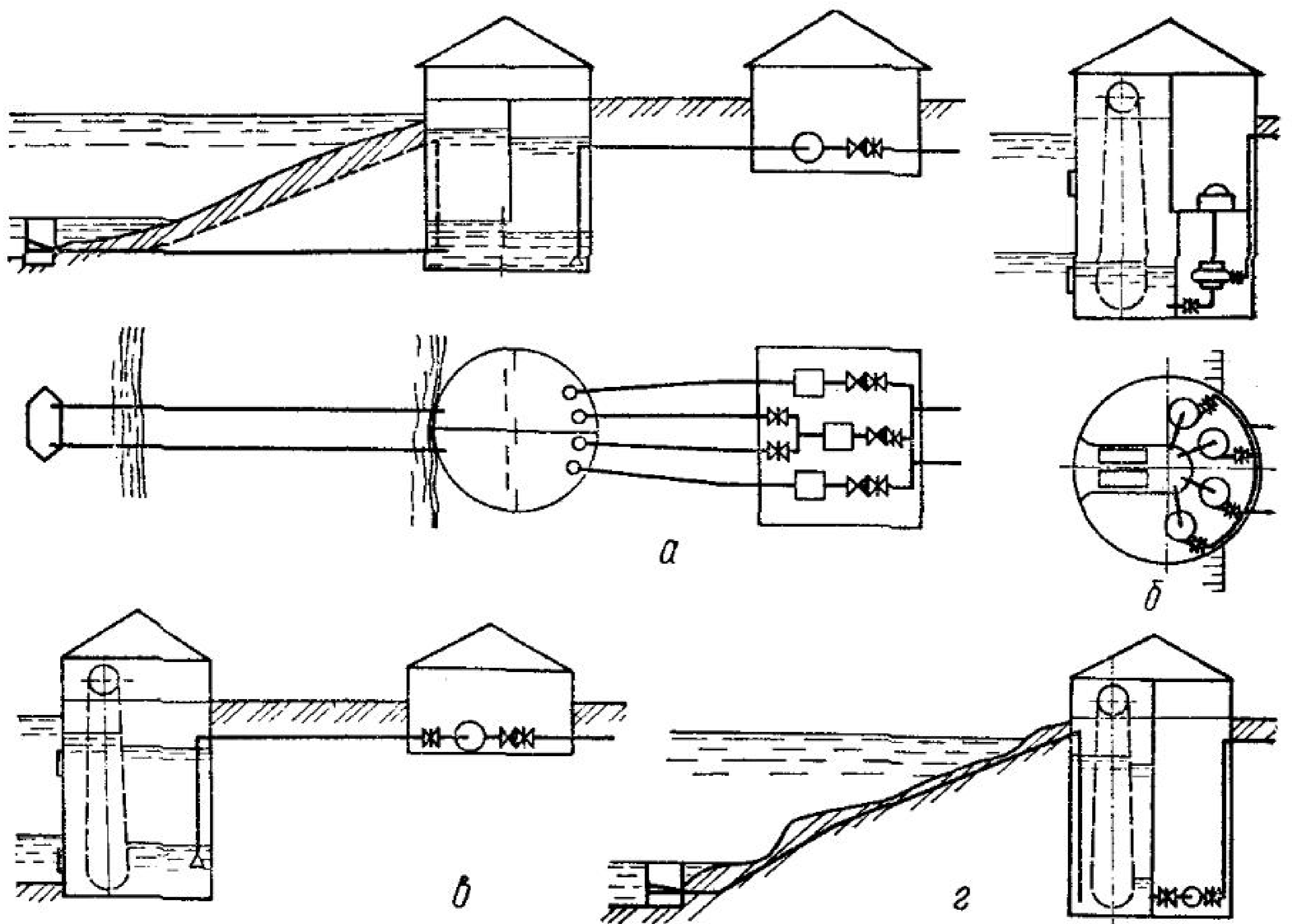
Рис. 39. Схемы насосных станций I подъема:
