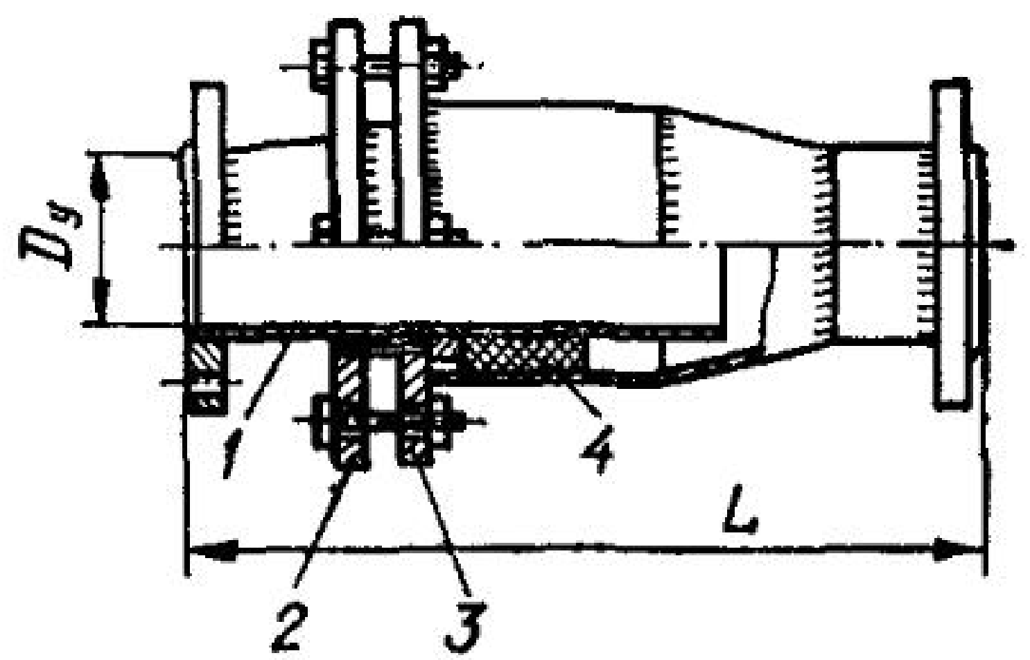
Рис. 21. Сальниковый компенсатор, используемый в качестве монтажной вставки:
