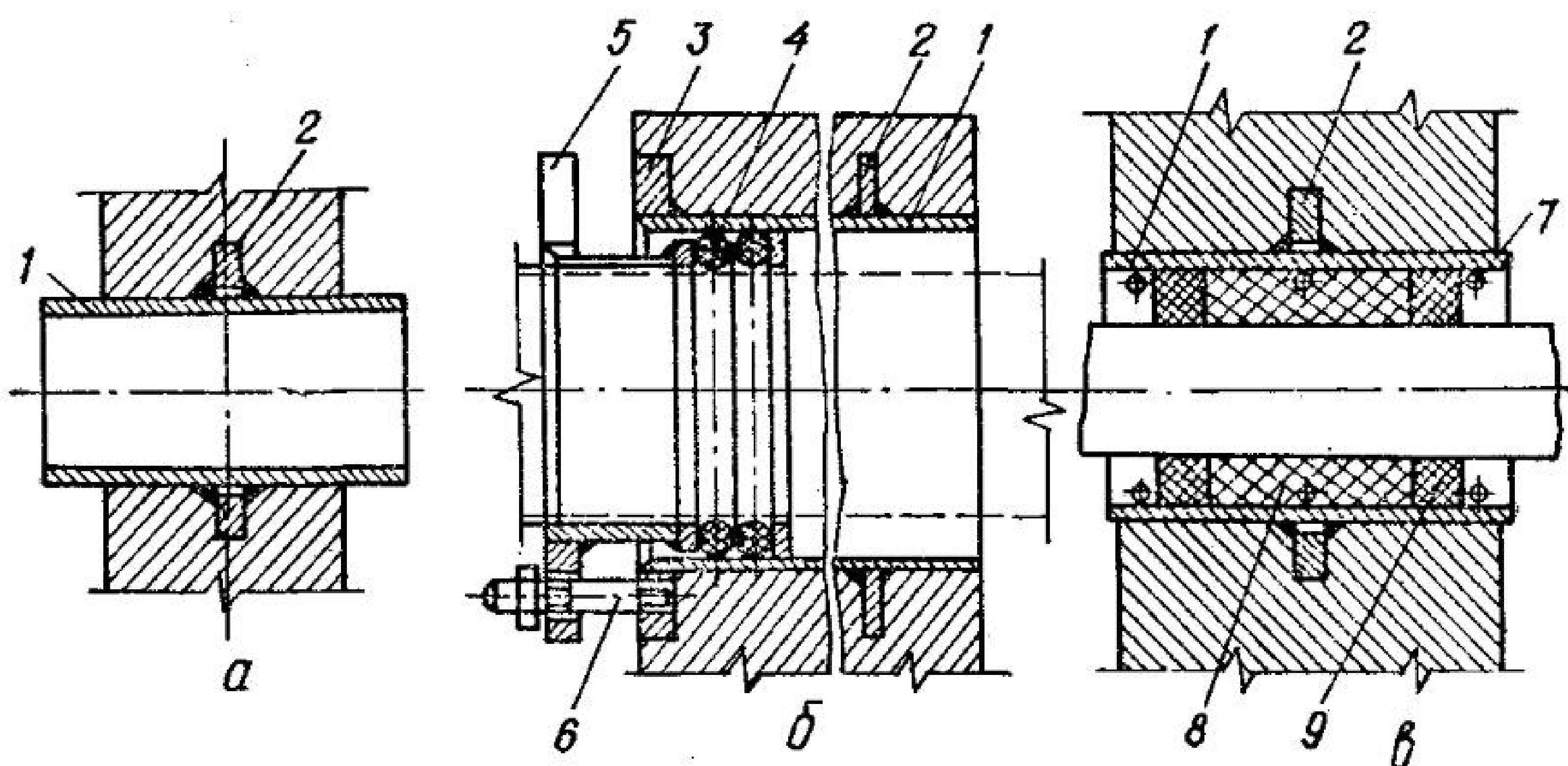
Рис. 16. Устройства для прохода трубопроводов через стену
