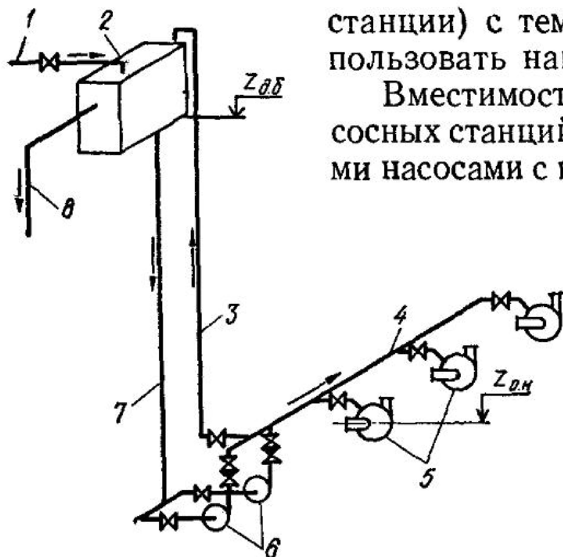
Рис. 63. Схема подачи воды для охлаждения и гидроуплотнения сальников канализационных насосов:
