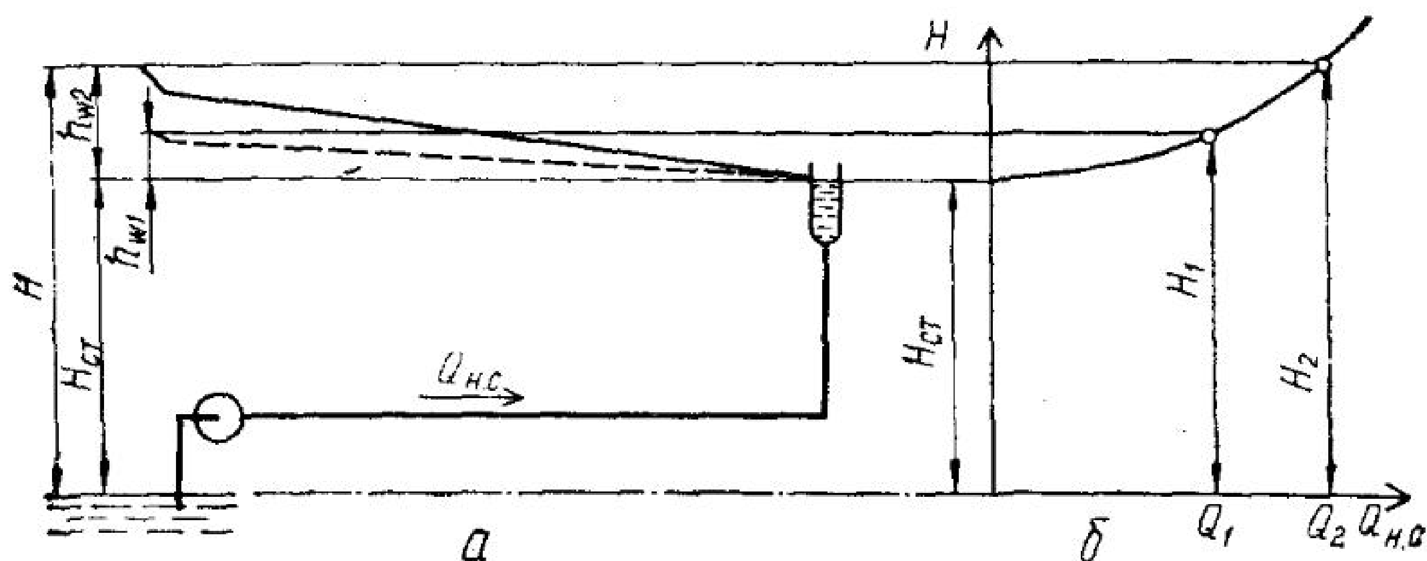
Рис. 23. К построению характеристики трубопровода: а — высотная схема; б — характеристика трубопровода
