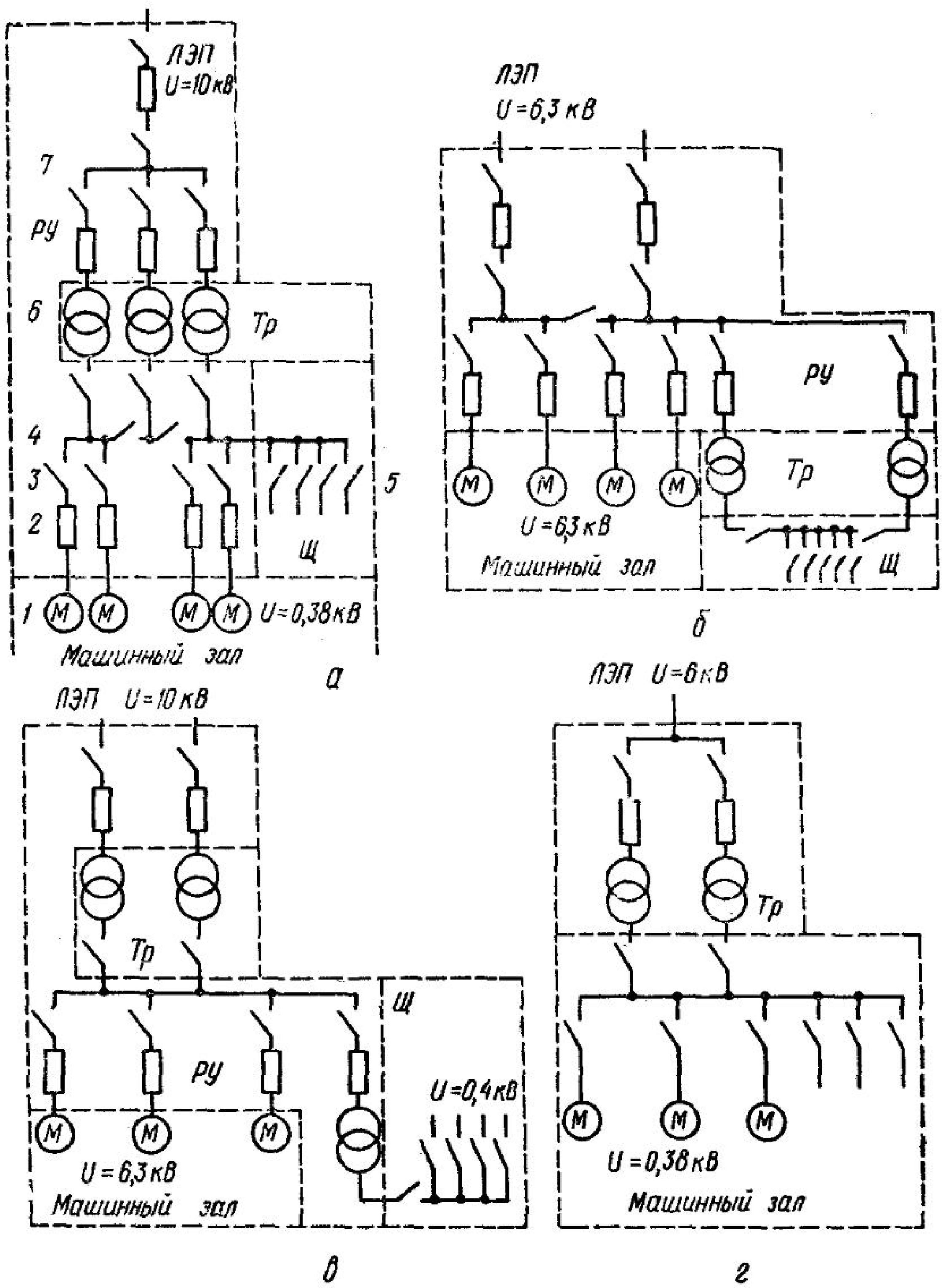
Рис. 36. Схемы электрических соединений насосных станций: а, б, в, г — различные варианты электрических соединений; 1 — электродвигатель насоса; 2 — масляный выключатель; 3 — разъединитель; 4 — шины низкого напряжения; 5 — щит низкого напряжения; б — силовой трансформатор; 7 — шины высокого напряжения; РУ — помещение распределительных устройств; Тр — камеры трансформаторов; Щ — щитовое помещение
