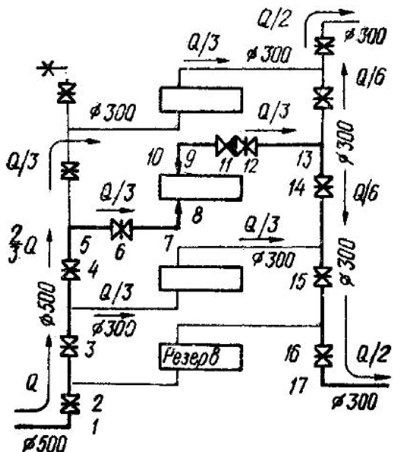
Рис. 25. Схема к определению потерь напора в насосной станции
