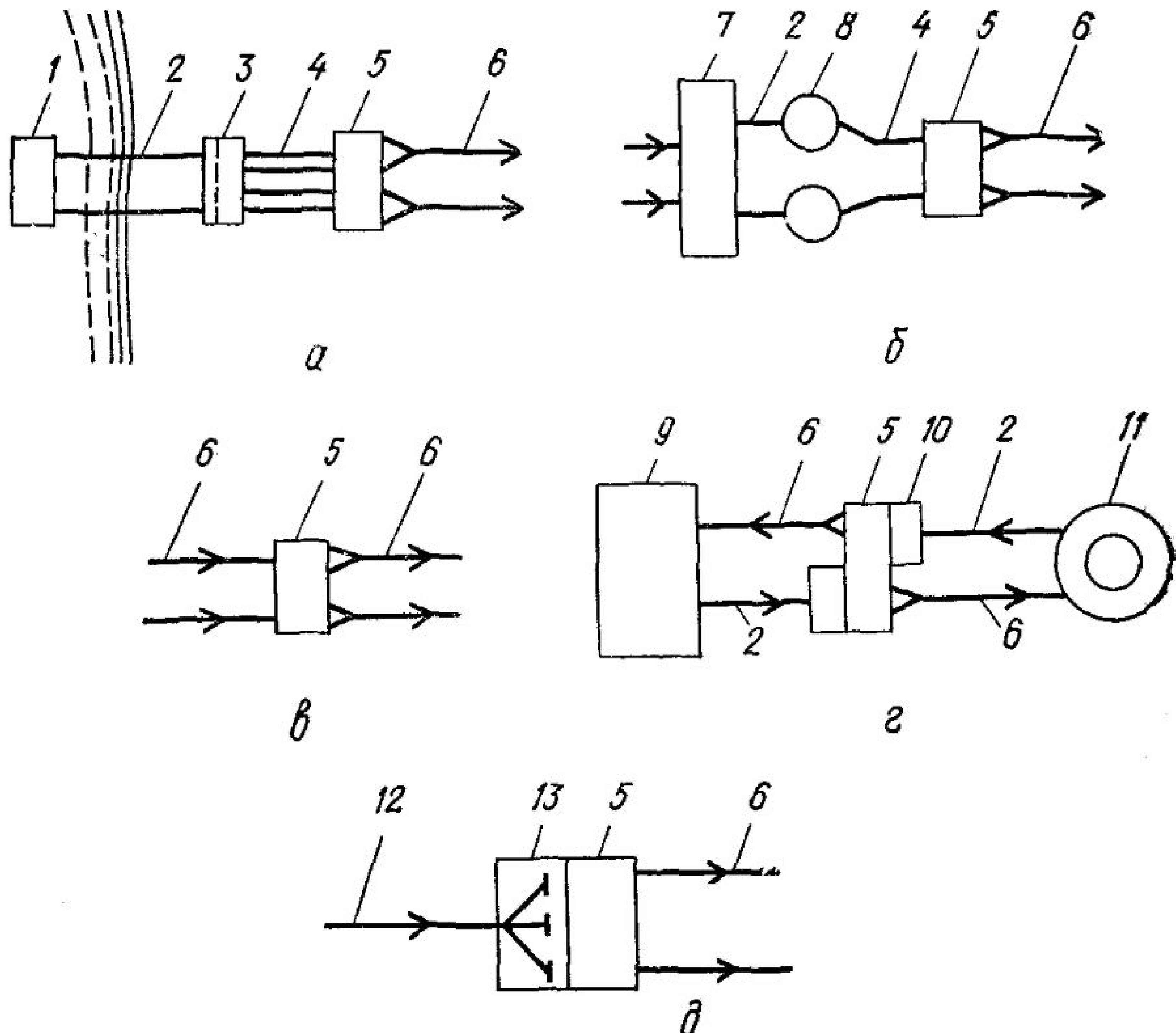
Рис. 1. Принципиальные схемы компоновки насосных станций различного назначения:
