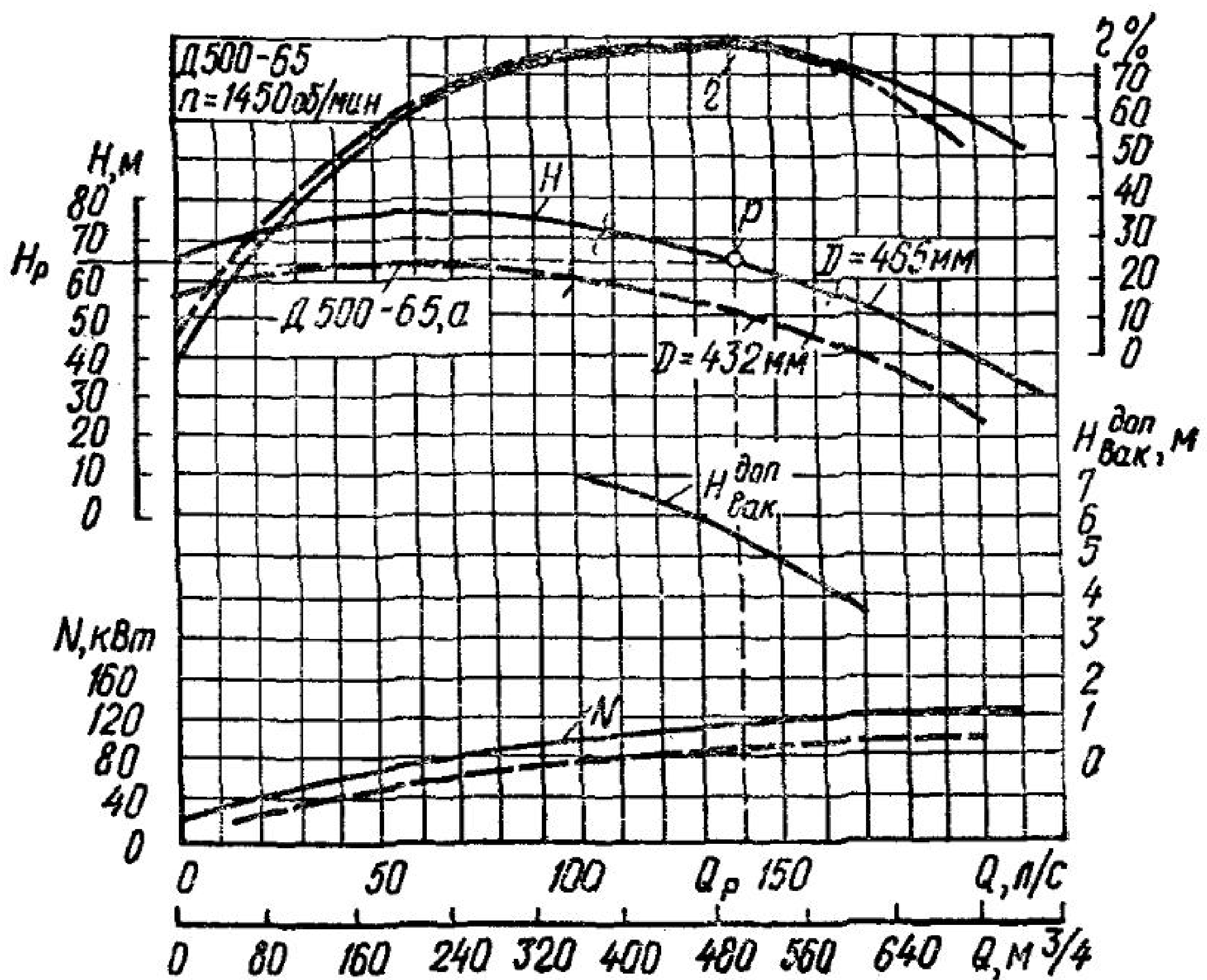
Рис. 2. Характеристики центробежного насоса
