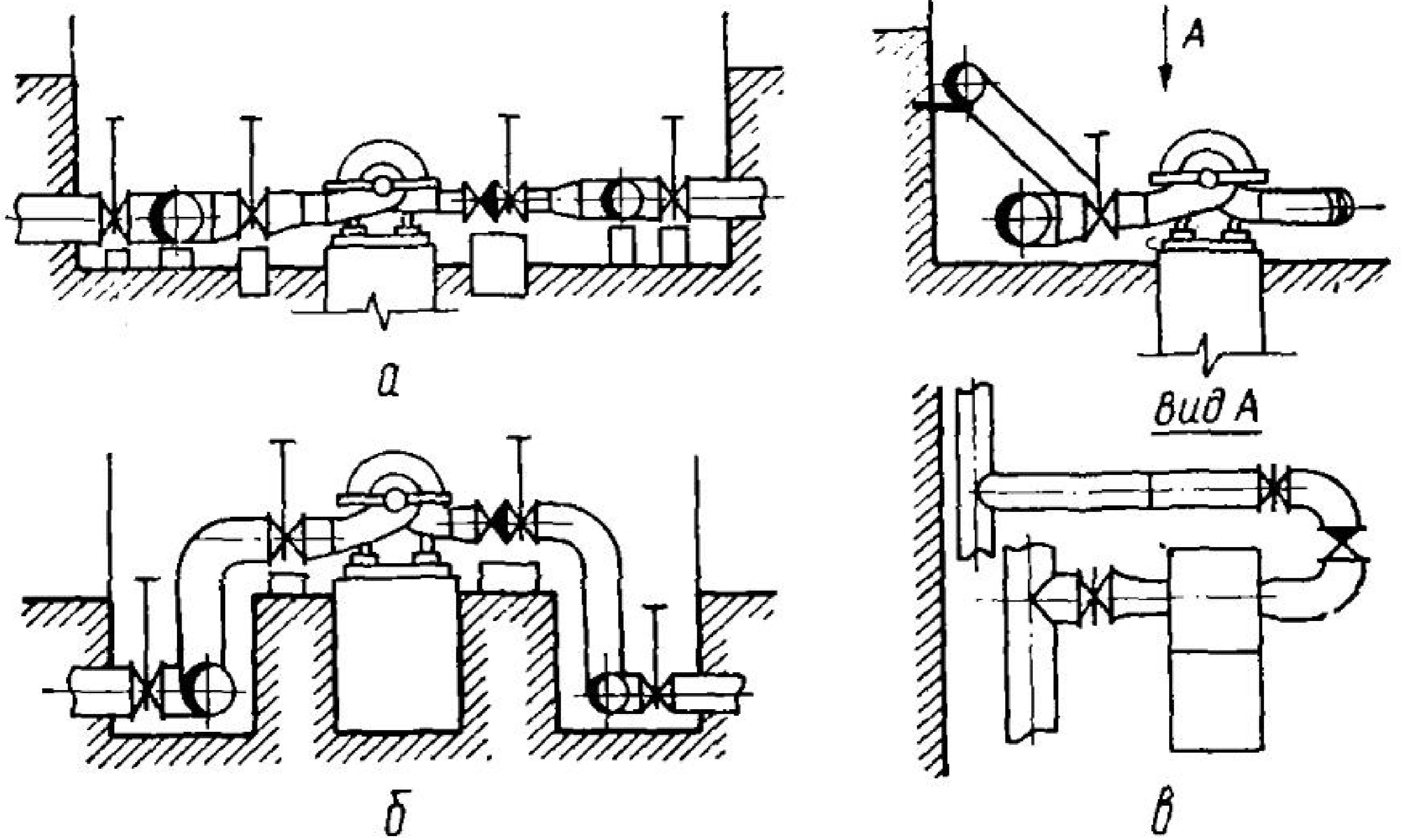
Рис. 56. Основные схемы размещения трубопроводов на станциях II подъема:
