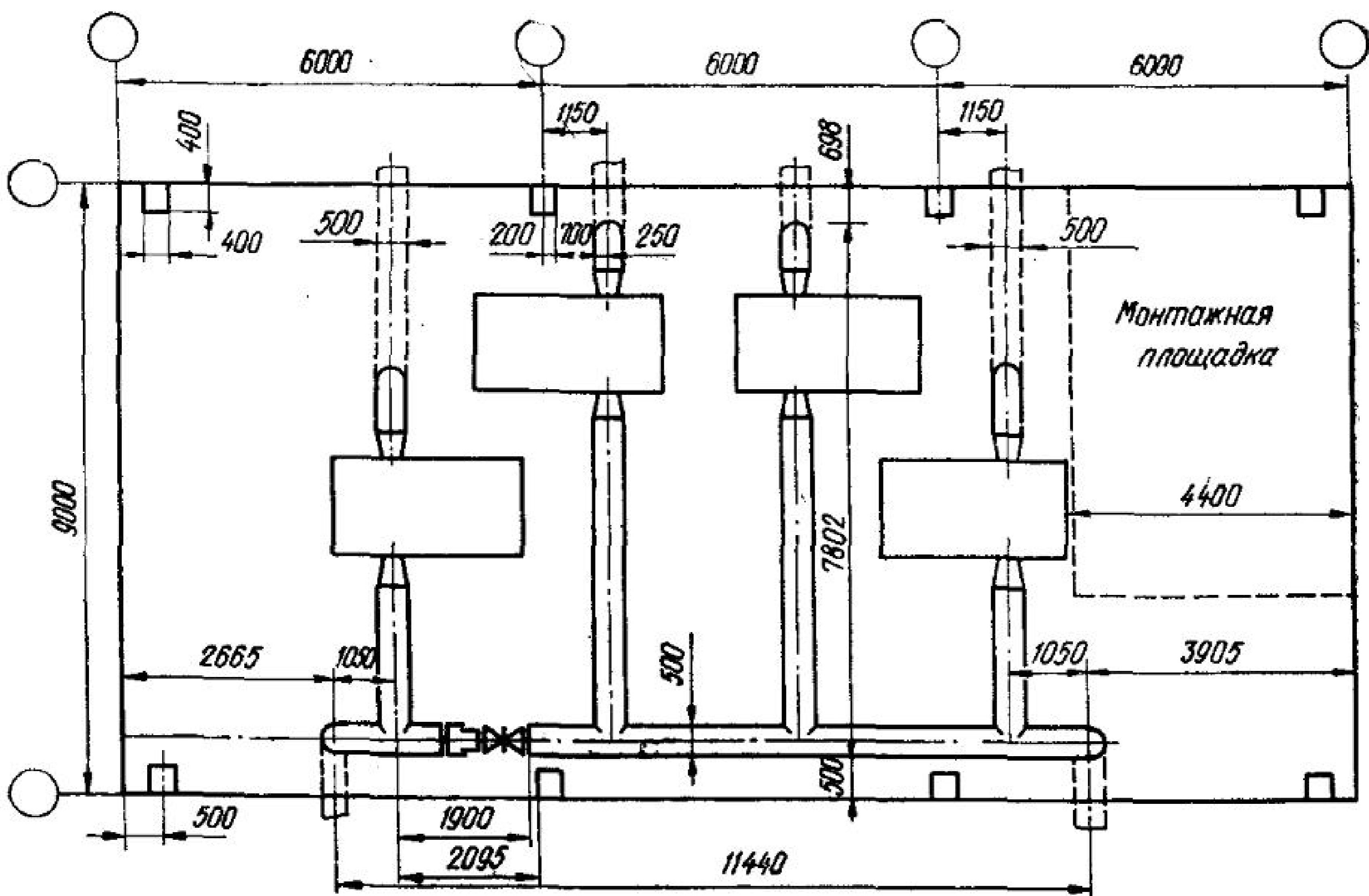
Рис. 47. Схема к определению размеров машинного зала с учетом сетки колонн
