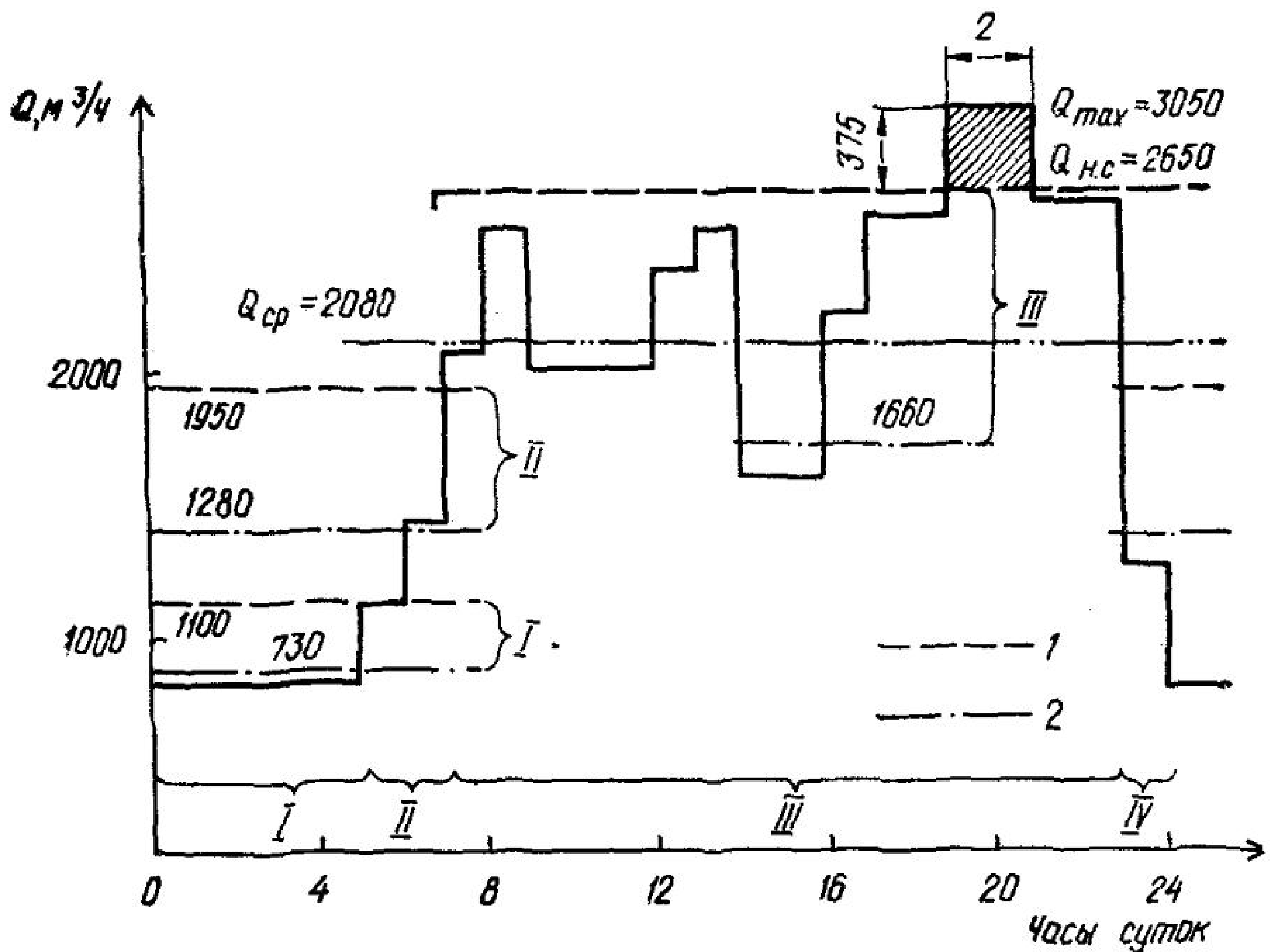
Рис. 48. Почасовой график водопотребления города и подачи насосной станции II подъема:
