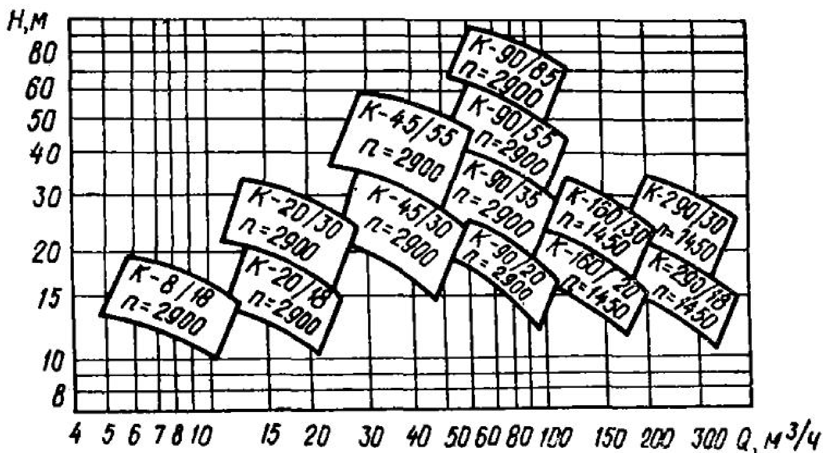
Рис. 4. Сводный график полей насосного типа К (КМ)
