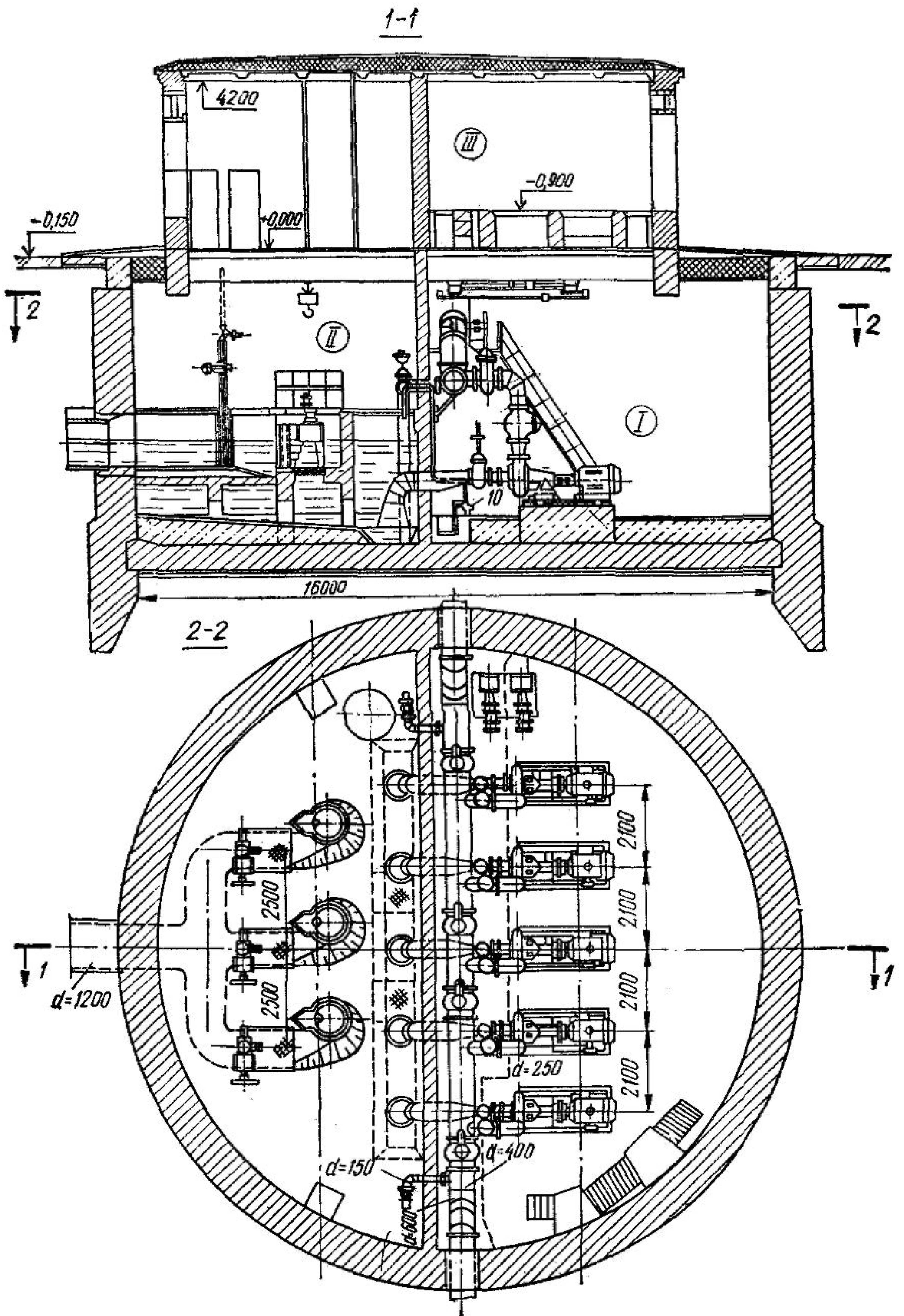
Рис. 60. Насосная станция водоотведения с горизонтальными насосами и решетками-дробилками: I — машинное отделение; II — приемный резервуар; III — верхнее строение
